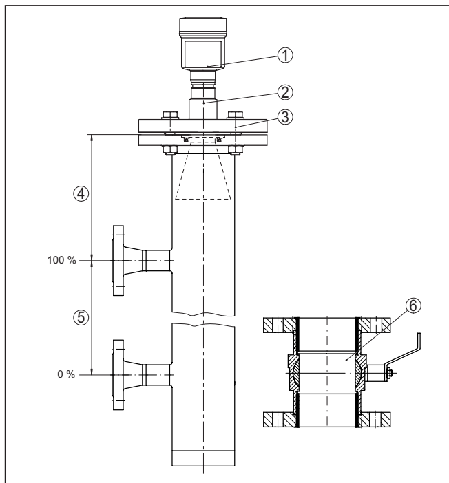
Рис. 15: Монтаж в выносной трубе
