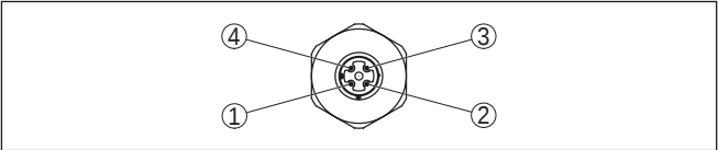
Рис. 24: Вид штекерного разъема
