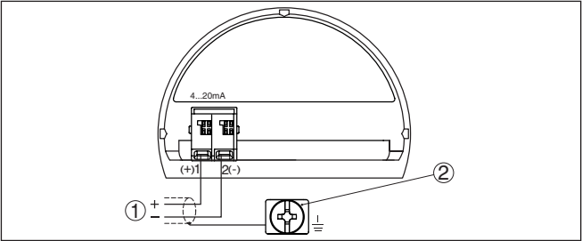
Рис. 23: Отсек подключения (двухкамерный корпус Ex d)
