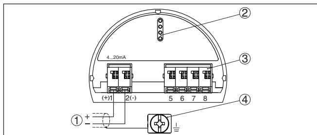
Рис. 18: Отсек электроники и подключения (однокамерный корпус)
