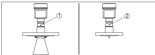
Рис. 5: Положение плоскости поляризации
