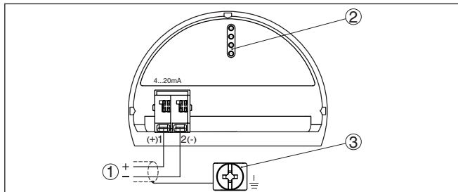
Рис. 20: Отсек подключения (двухкамерный корпус)
