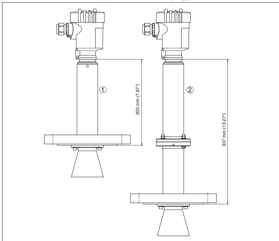
Рис. 59: VEGAPULS 66, исполнение для высоких температур
