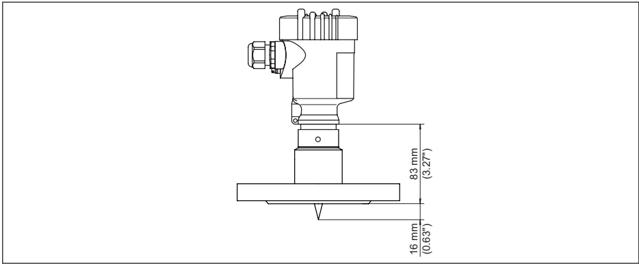
Рис. 58: VEGAPULS 66, исполнение без рупорной антенны
