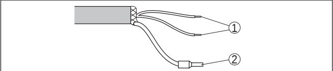
Рис. 25: Назначение проводов постоянно подключенного соединительного кабеля
