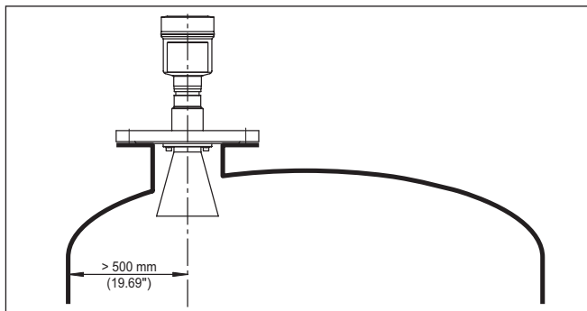
Рис. 6: Монтаж на выпуклой крыше емкости
