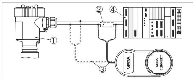
Рис. 31: Подключение ПК к сигнальному кабелю через HART
