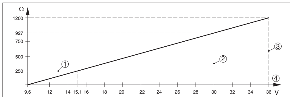
Рис. 50: Диаграмма напряжения
