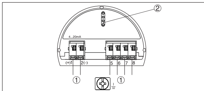
Рис. 19: Отсек электроники (двухкамерный корпус)
