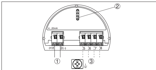
Рис. 22: Отсек электроники (двухкамерный корпус)
