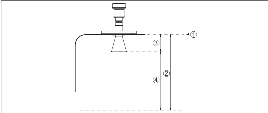
Рис. 48: Данные для входной величины
