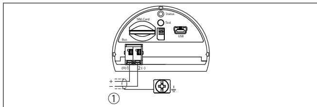
Рис. 21: Подключение модуля мобильной связи к питанию
