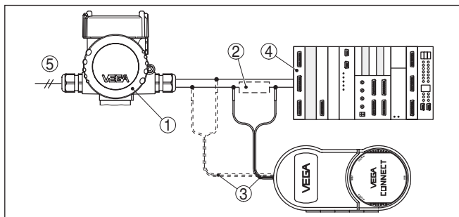
Рис. 26: Подключение ПК к сигнальному кабелю через HART
