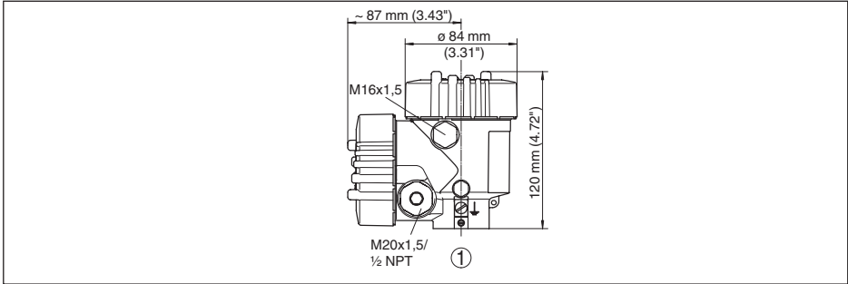
Рис. 45: Размеры корпуса - с установленным модулем индикации и настройки корпус выше на 9 мм (0.35 in)
