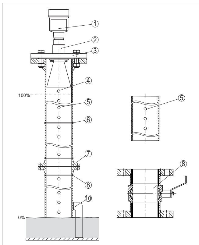
Рис. 14: Монтаж в уравнильной трубе
