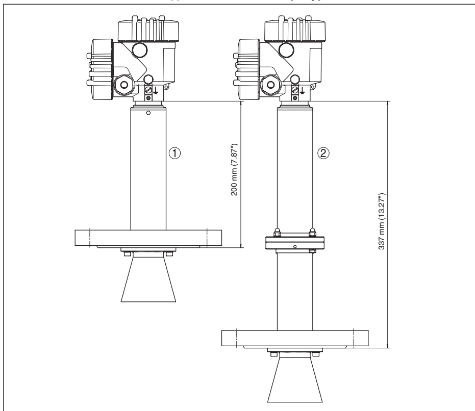
Рис. 48: VEGAPULS 66, исполнение для высоких температур
