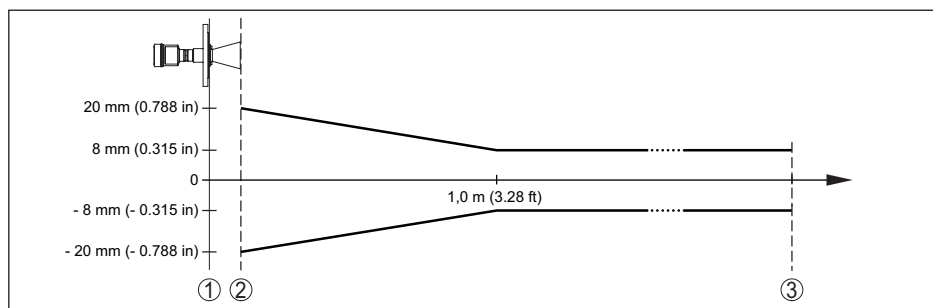
Рис. 44: Погрешность измерения при эталонных условиях
