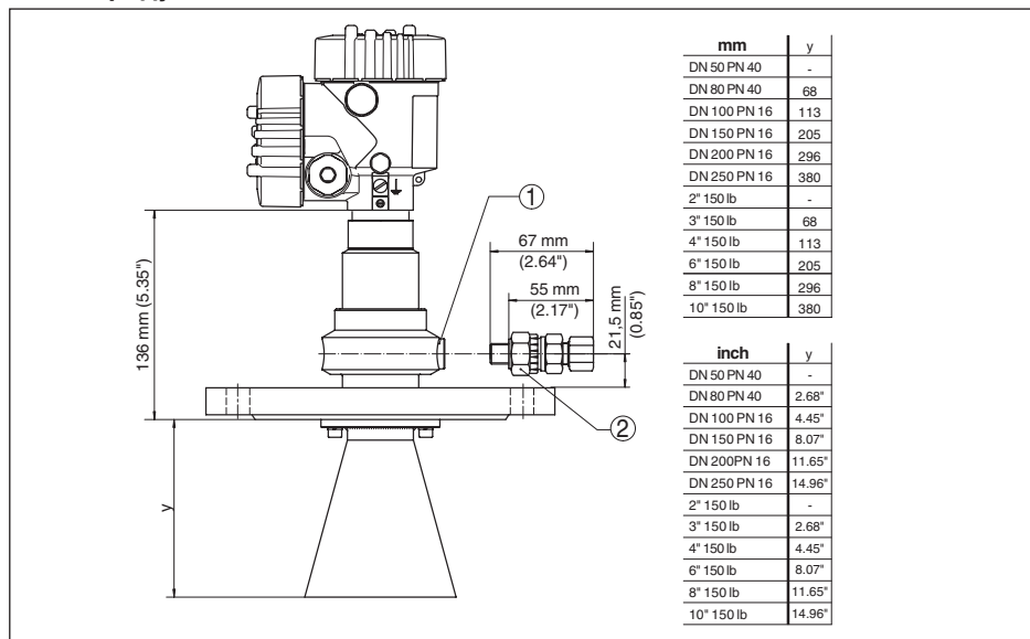
Рис. 47: VEGAPULS 66, стандартное исполнение со входом для подключения продувки
