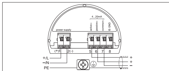
Рис. 18: Отсек подключения в двухкамерном корпусе в случае сетевого напряжения
