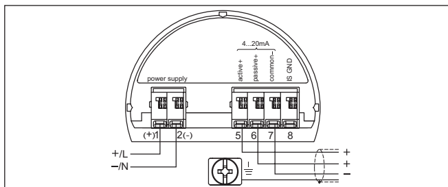
Рис. 19: Отсек подключения в двухкамерном корпусе в случае малого напряжения
