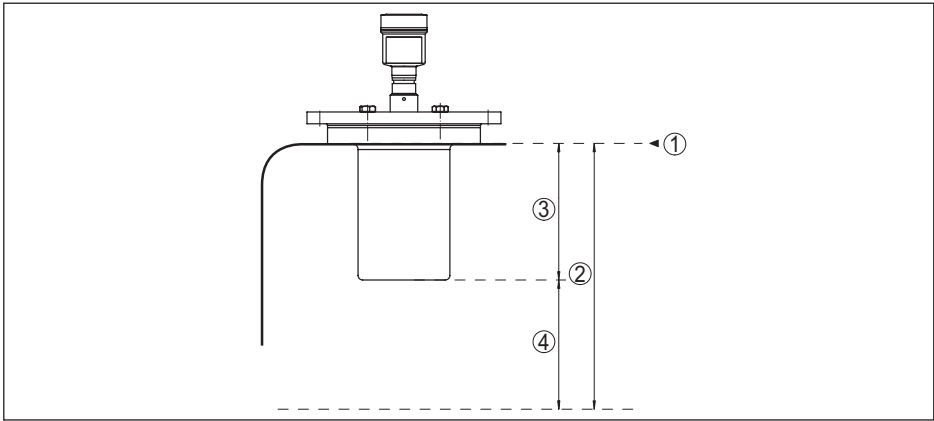
Рис. 42: Данные для входной величины
