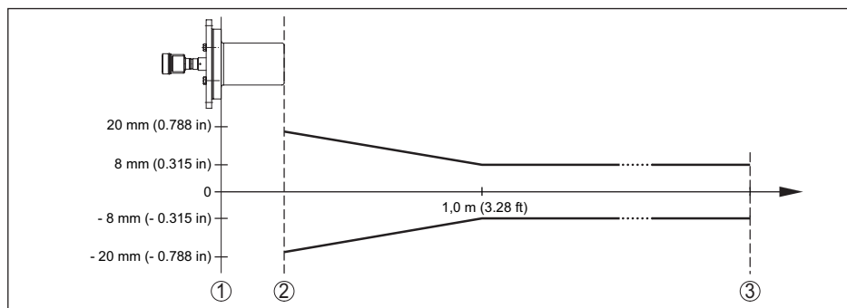
Рис. 43: Погрешность измерения при эталонных условиях
