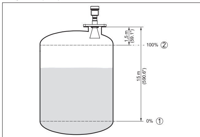
Рис. 23: Пример выполнения Установки Min./Max.
