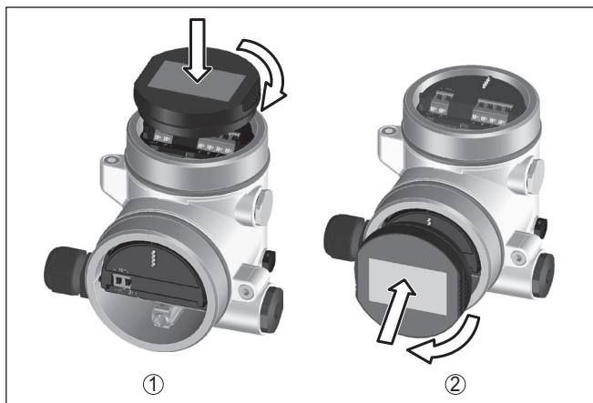
Рис. 21: Установка модуля индикации и настройки в двухкамерном корпусе
