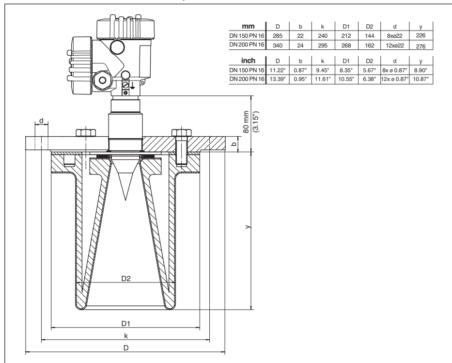
Рис. 45: VEGAPULS 66 с эмалевым покрытием
