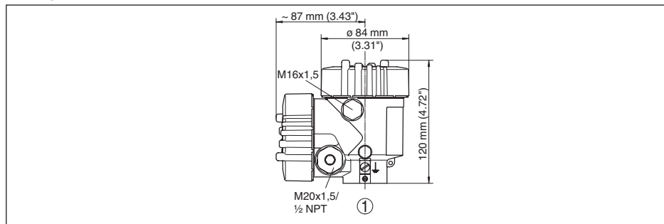
Рис. 44: Размеры корпуса - с установленным модулем индикации и настройки корпус выше на 9 мм (0.35 in)
