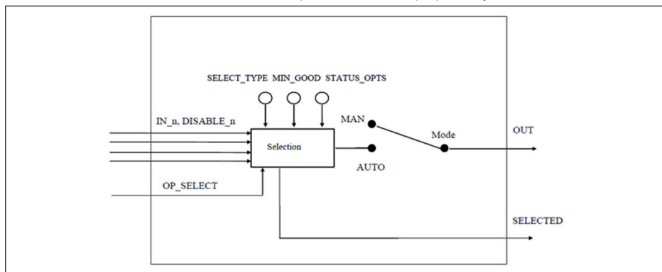
Рис. 55: Схема функционального блока Input Selector
