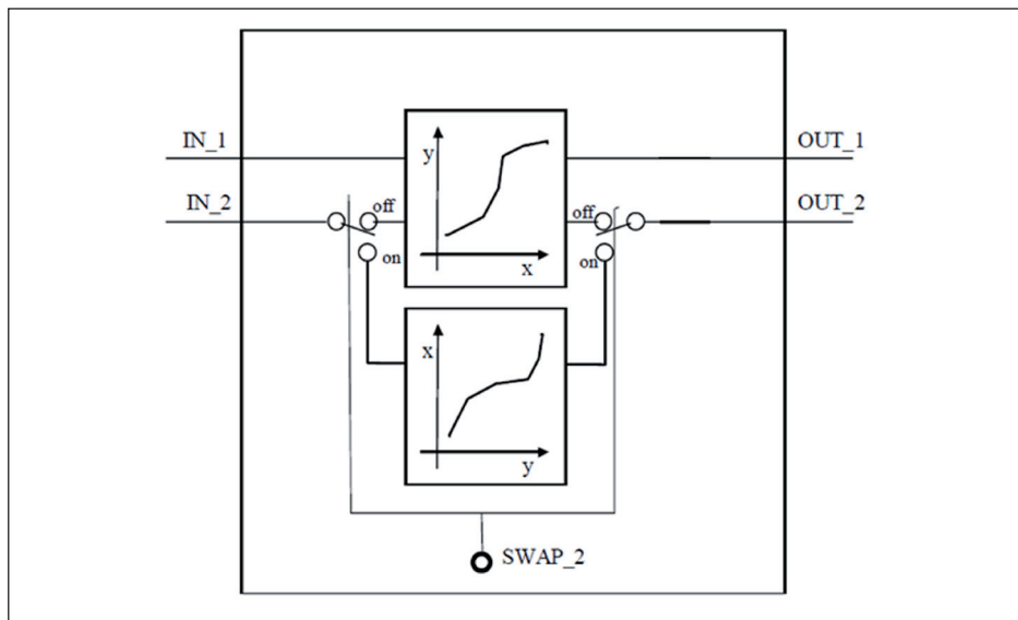
Рис. 53: Схема функционального блока Signal Characterizer
