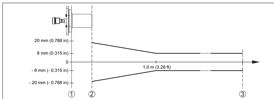
Рис. 47: Погрешность измерения при эталонных условиях
