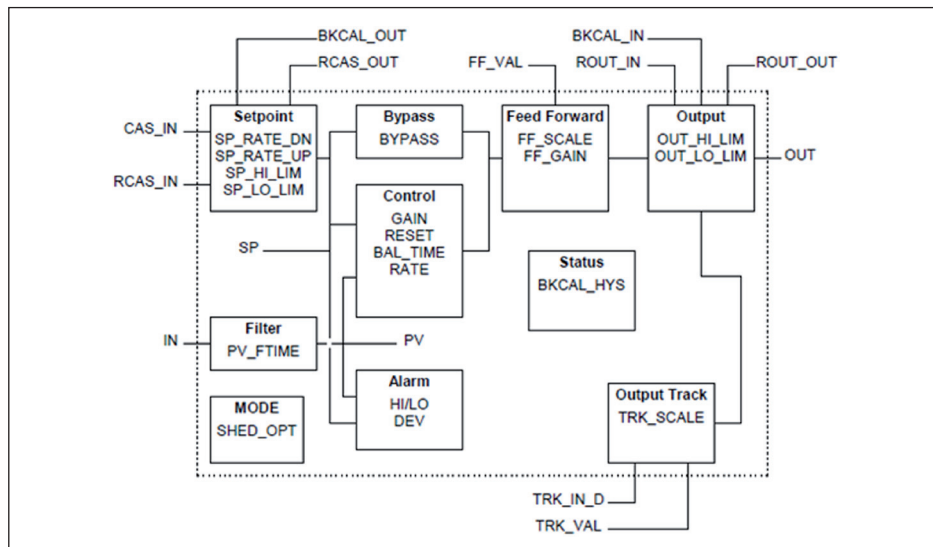
Рис. 51: Схема функционального блока PID Control
