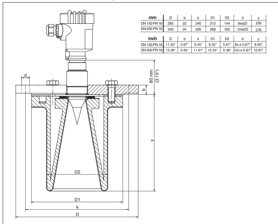
Рис. 62: VEGAPULS 66 с эмалевым покрытием
