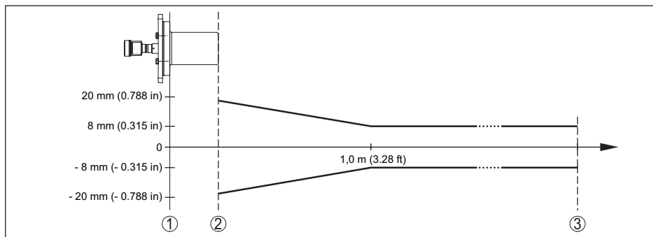
Рис. 45: Погрешность измерения при эталонных условиях
