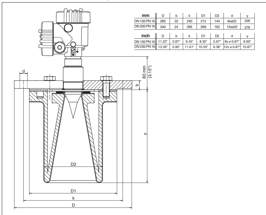
Рис. 53: VEGAPULS 66 с эмалевым покрытием
