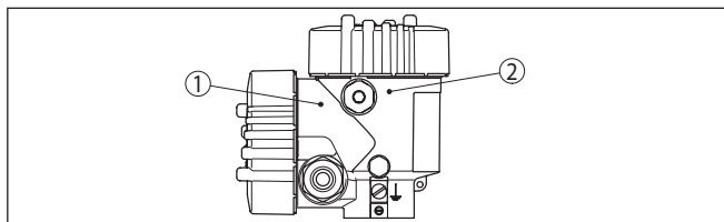
Рис. 18: Позиция отсека подключения (электроника Modbus) и отсека электроники (электроника датчика)
