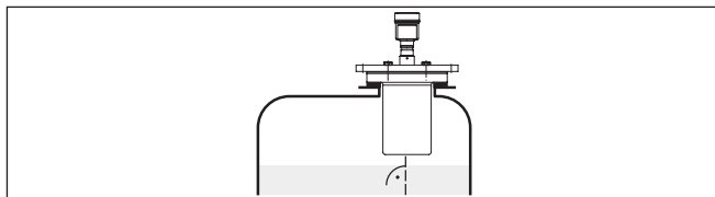
Рис. 11: Ориентация датчика на жидкостях
