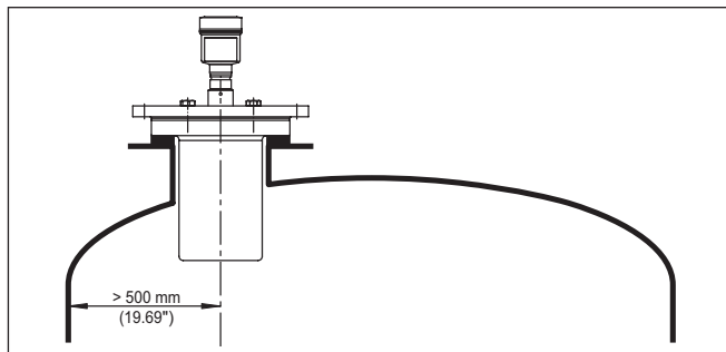
Рис. 7: Монтаж радарного датчика на округлой крыше емкости
