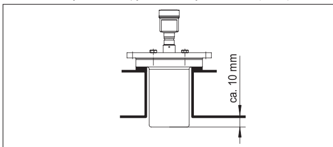
Рис. 10: Рекомендуемая высота монтажного патрубка
