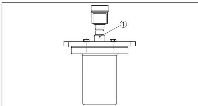
Рис. 6: Положение плоскости поляризации
