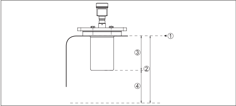
Рис. 44: Данные для входной величины
