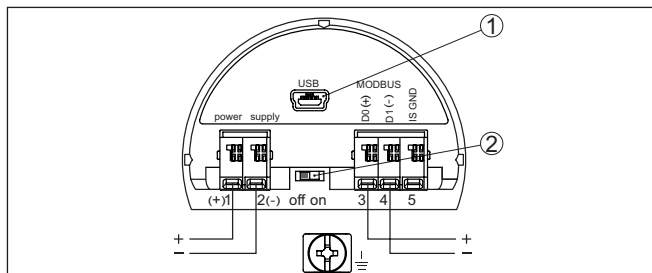
Рис. 20: Отсек подключения
