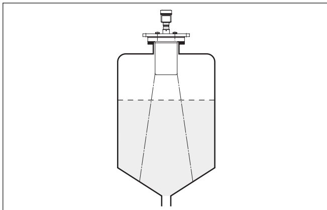
Рис. 8: Монтаж радарного датчика на емкостях с коническим дном
