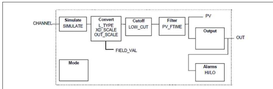
Рис. 50: Схема функционального блока Analog Input (AI)
