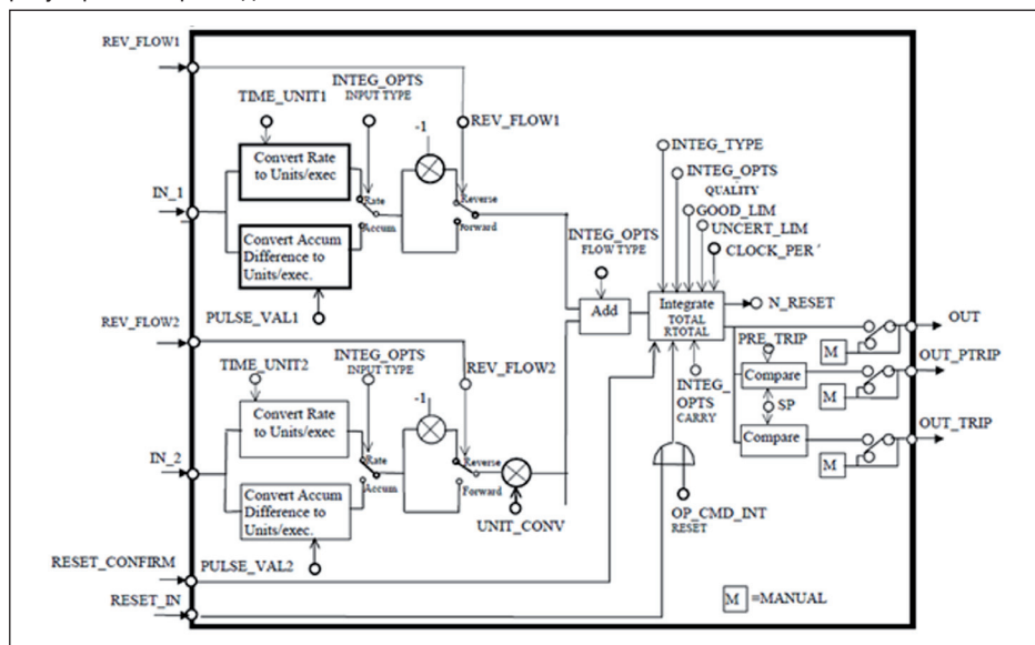
Рис. 55: Схема функционального блока Integrator
