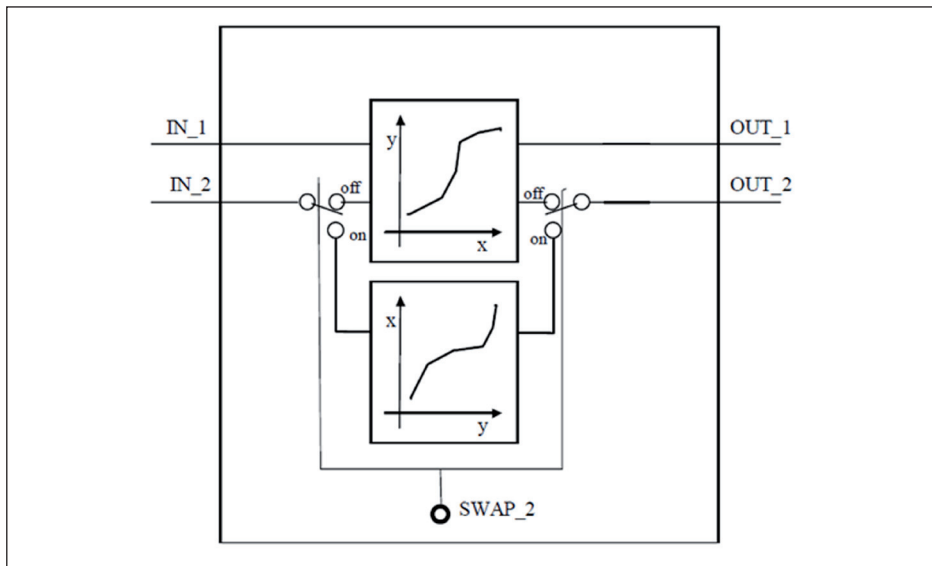
Рис. 54: Схема функционального блока Signal Characterizer
