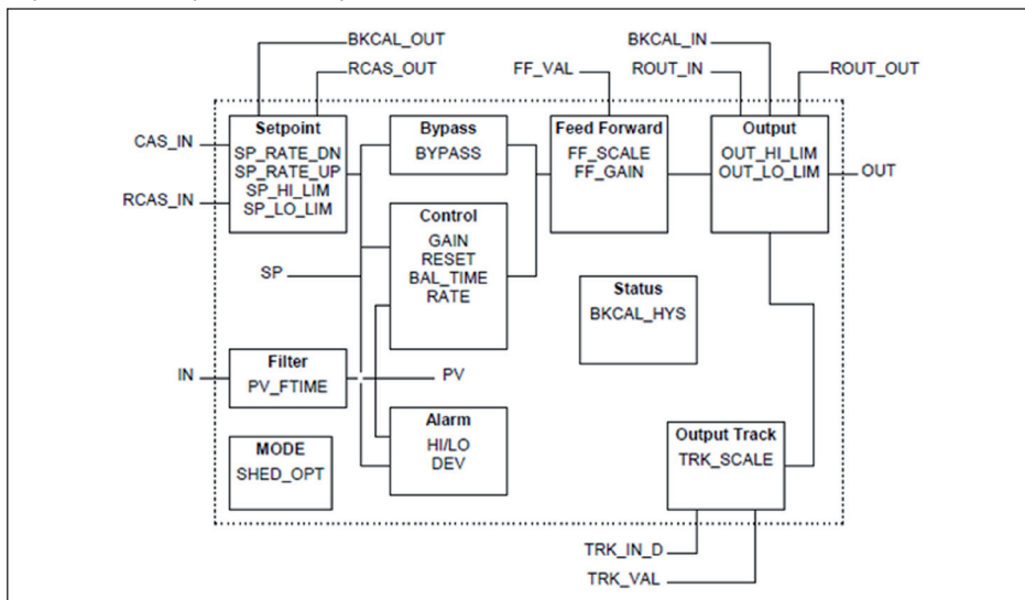
Рис. 52: Схема функционального блока PID Control
