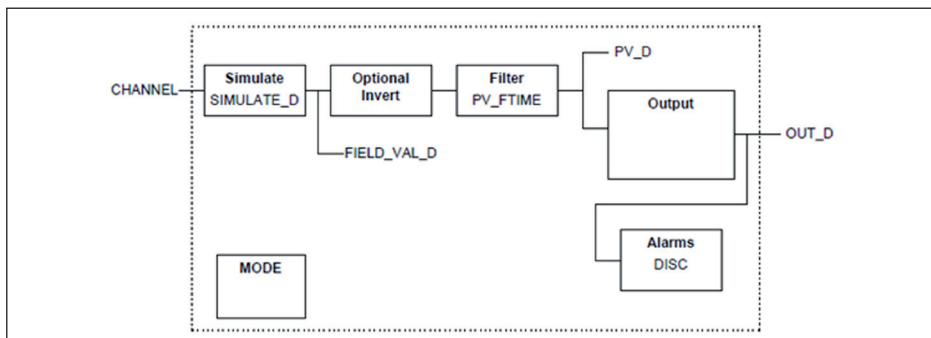
Рис. 51: Схема функционального блока Discret Input (DI)
