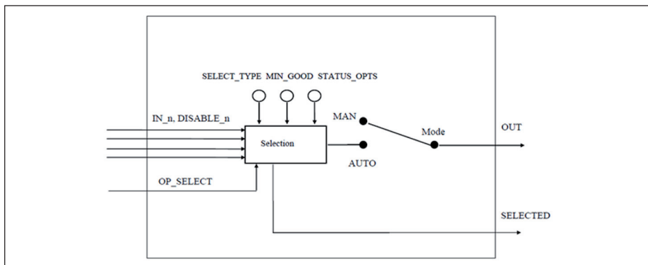
Рис. 56: Схема функционального блока Input Selector
