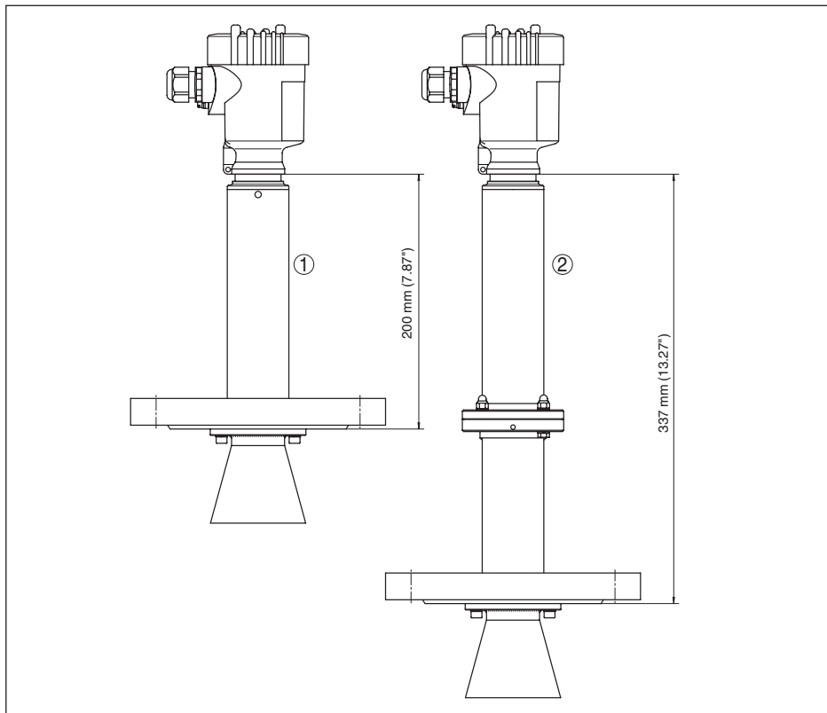
Рис. 66: VEGAPULS 66, исполнение для высоких температур
