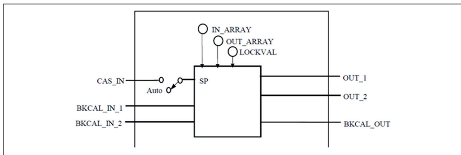
Рис. 53: Схема функционального блока Output Splitter
