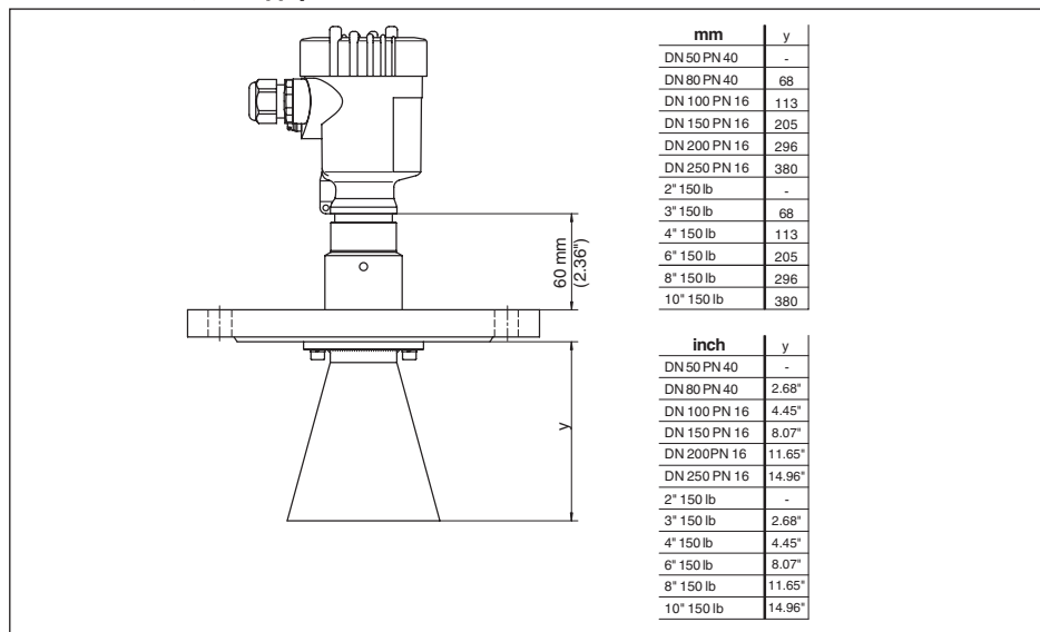
Рис. 63: VEGAPULS 66, стандартное исполнение
