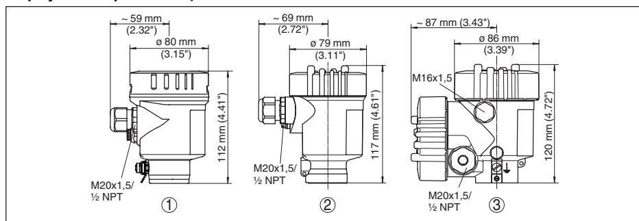
Рис. 61: Корпуса в исполнении IP 66/IP 68 (0,2 bar) - с установленным модулем индикации и настройки корпус выше на 9 mm/0.35 in
