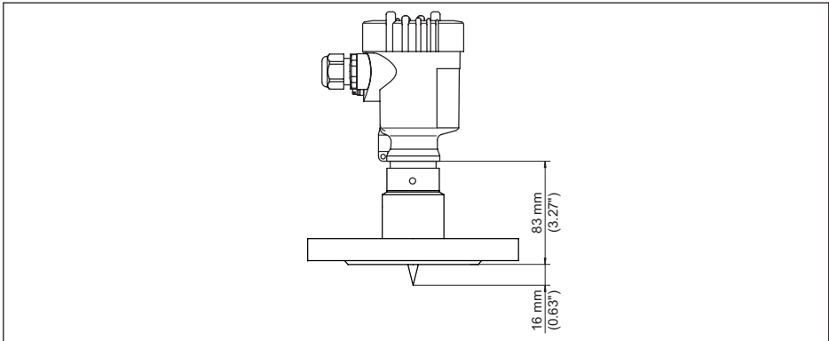
Рис. 65: VEGAPULS 66, исполнение без рупорной антенны
