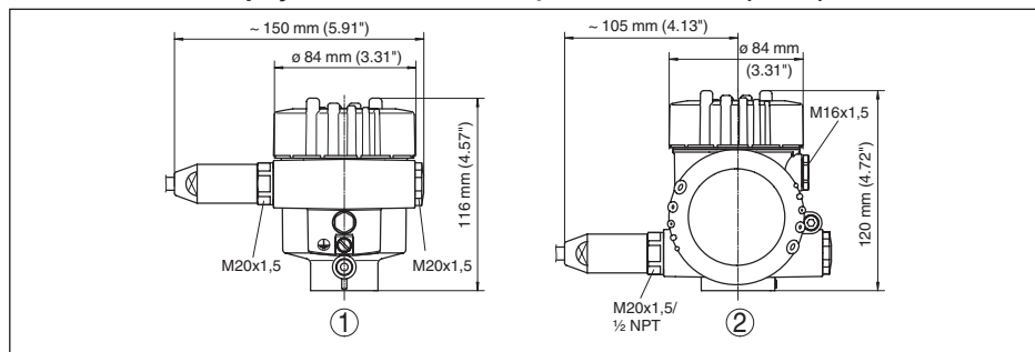
Рис. 60: Корпуса в исполнении IP 66/IP 68 (1 bar) - с установленным модулем индикации и настройки корпус выше на 9 mm/0.35 in
