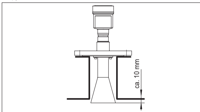
Рис. 11: Удлинительная труба
