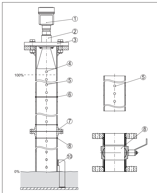
Рис. 15: Монтаж в уравнительной трубе
