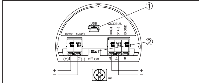
Рис. 21: Отсек подключения
