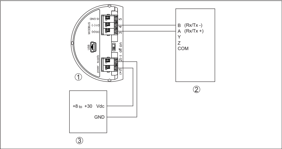
Рис. 47: Подключение VEGAPULS 66 к RTU Fisher ROC 809
