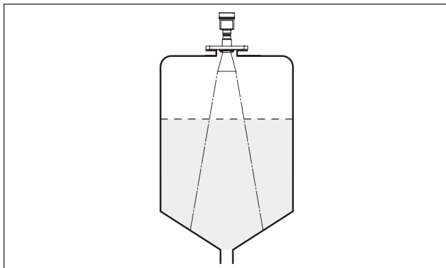
Рис. 8: Емкость с коническим дном
