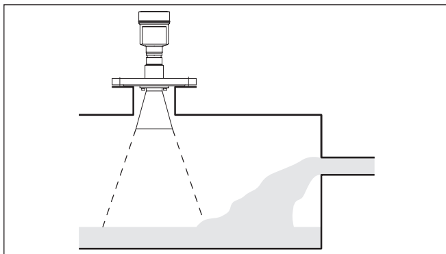
Рис. 9: Монтаж радарного датчика при втекающем продукте
