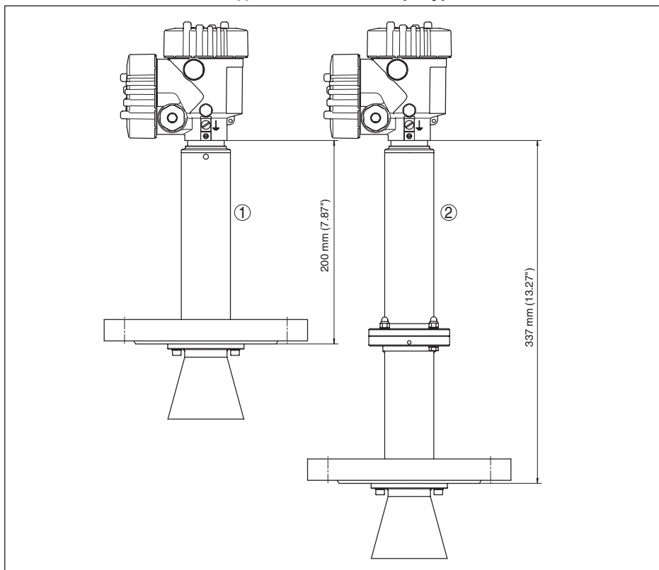
Рис. 55: VEGAPULS 66, исполнение для высоких температур
