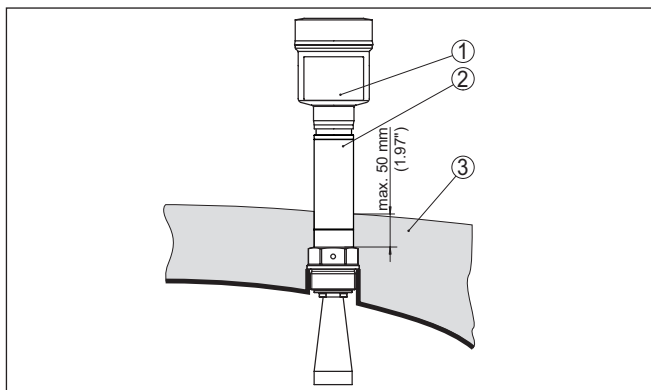
Рис. 17: Монтаж устройства на емкости с термоизоляцией
