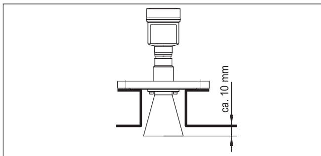
Рис. 10: Рекомендуемая высота монтажного патрубка
