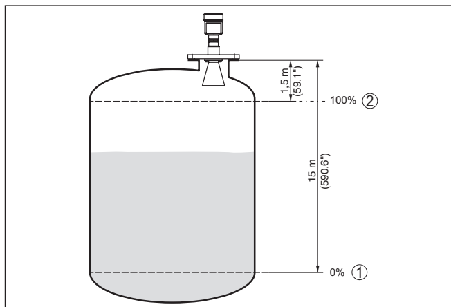
Рис. 24: Пример выполнения Установки Min./Max.
