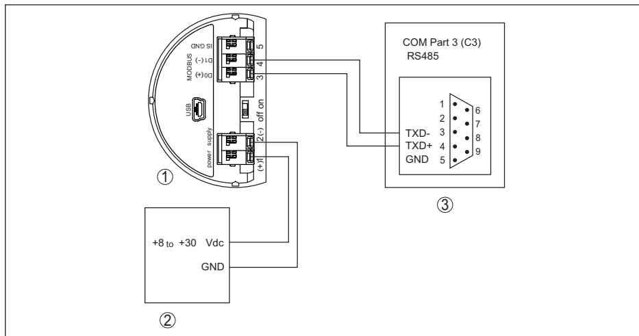
Рис. 51: Подключение VEGAPULS 66 к RTU ScadaPack
