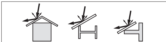
Рис. 13: Отражатели над конструкциями в емкости
