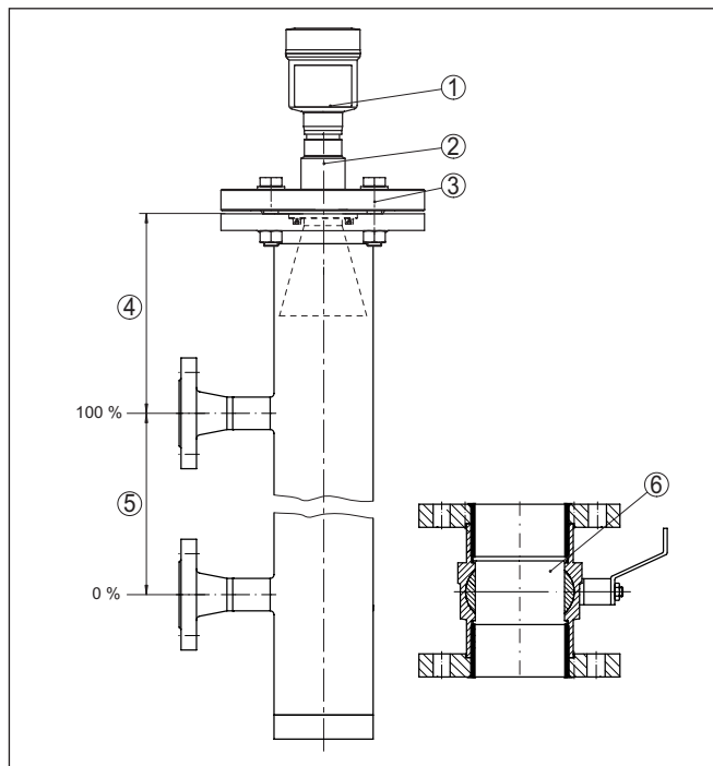
Рис. 16: Монтаж в выносной трубе
