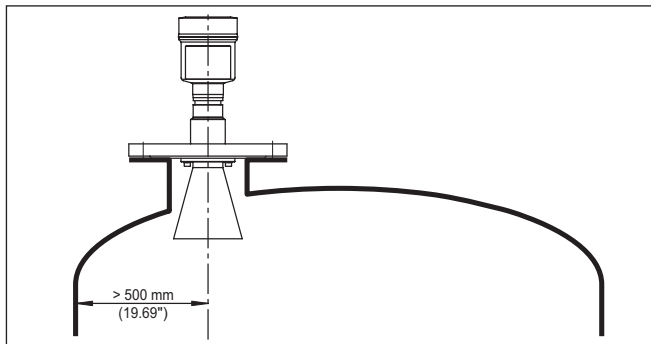
Рис. 7: Монтаж на выпуклой крыше емкости
