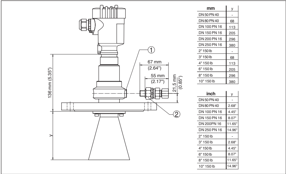
Рис. 59: VEGAPULS 66, стандартное исполнение со входом для подключения продувки
