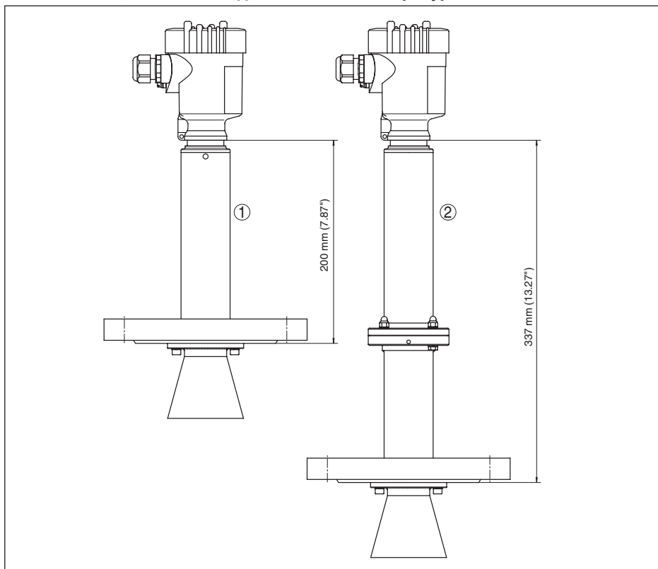
Рис. 61: VEGAPULS 66, исполнение для высоких температур
