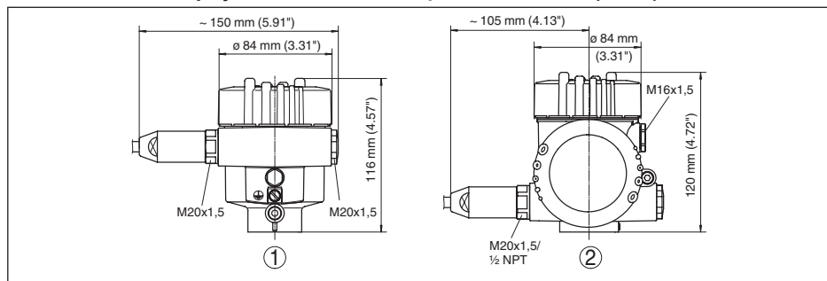
Рис. 55: Корпуса в исполнении IP 66/IP 68 (1 bar) - с установленным модулем индикации и настройки корпус выше на 9 mm/0.35 in
