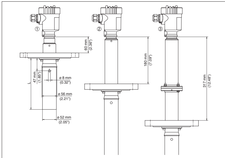
Рис. 37: VEGAPULS 66, исполнение с опускной трубой 5)
