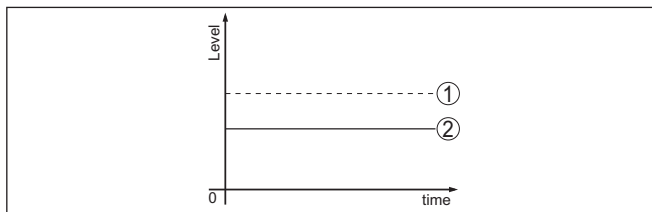
Рис. 20: Пунктирная линия 1 показывает действительный уровень, сплошная линия 2 показывает выдаваемый датчиком уровень
