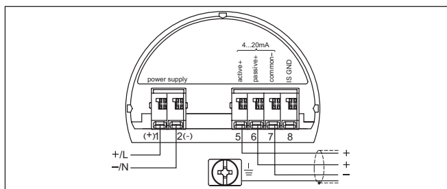
Рис. 29: Отсек подключения в двухкамерном корпусе в случае малого напряжения
