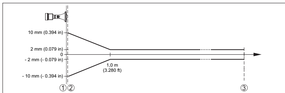
Рис. 48: Погрешность измерения при эталонных условиях
