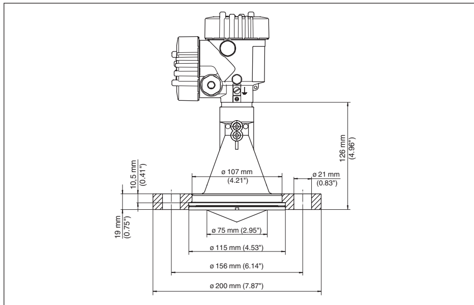
Рис. 51: VEGAPULS 67, накидной фланец для DN 80 PN 16/ ASME 3" 150lbs/ JIS80 10K
