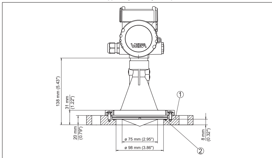
Рис. 52: VEGAPULS 67, адаптерный фланец
