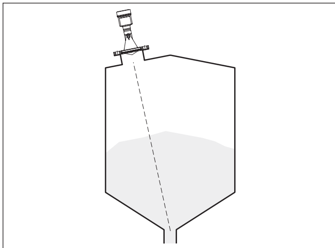
Рис. 15: Ориентация прибора в силосе
