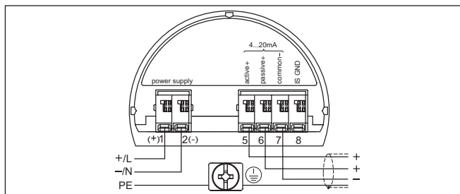
Рис. 28: Отсек подключения в двухкамерном корпусе в случае сетевого напряжения
