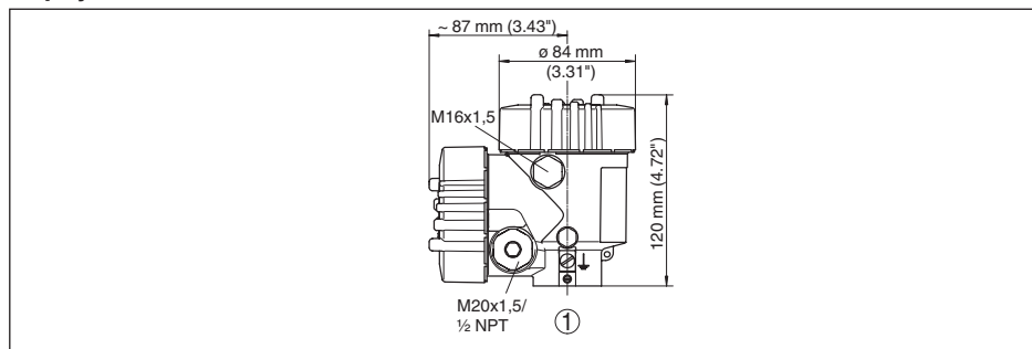
Рис. 49: Размеры корпуса - с установленным модулем индикации и настройки корпус выше на 9 мм (0.35 in)
