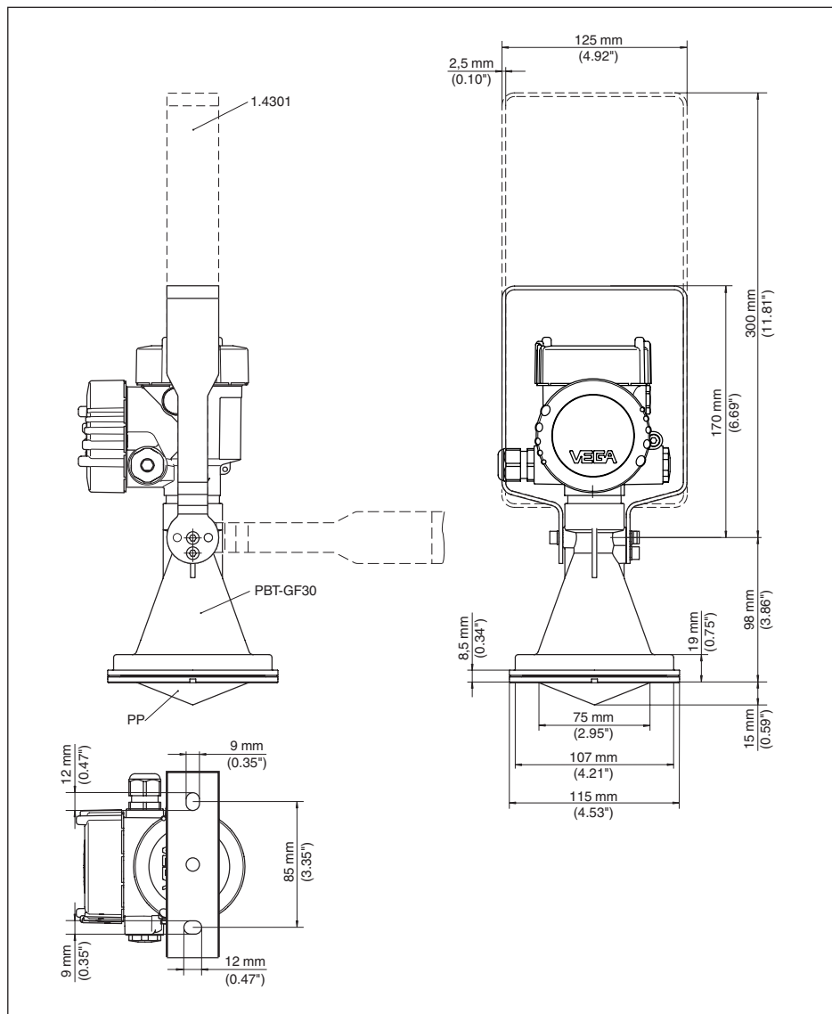
Рис. 50: VEGAPULS 67, с монтажной скобой
