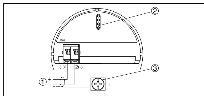
Рис. 14: Отсек подключения (двухкамерный корпус)
