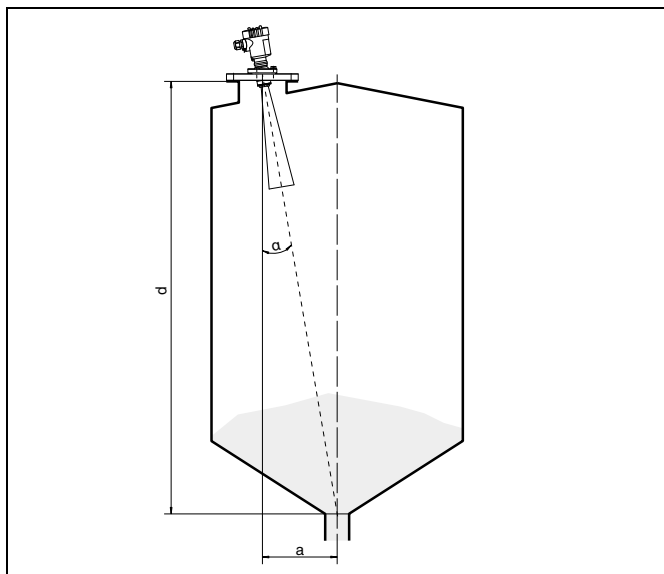
Рис. 5: VEGAPULS 68 с поворотным креплением
