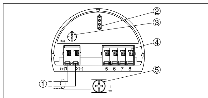
Рис. 13: Отсек электроники и подключения - однокамерный корпус
