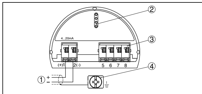
Рис. 8: Отсек электроники и подключения - однокамерный корпус
