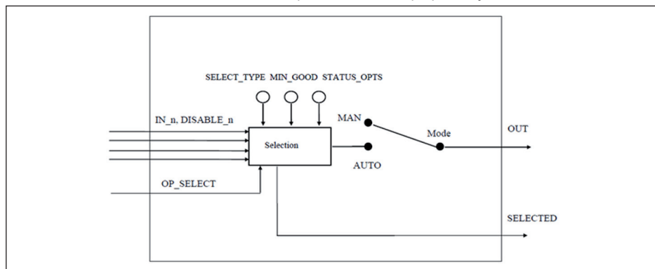
Рис. 60: Схема функционального блока Input Selector
