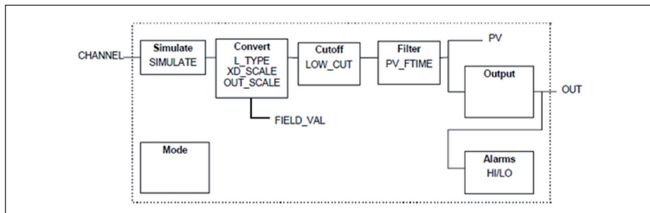
Рис. 54: Схема функционального блока Analog Input (AI)
