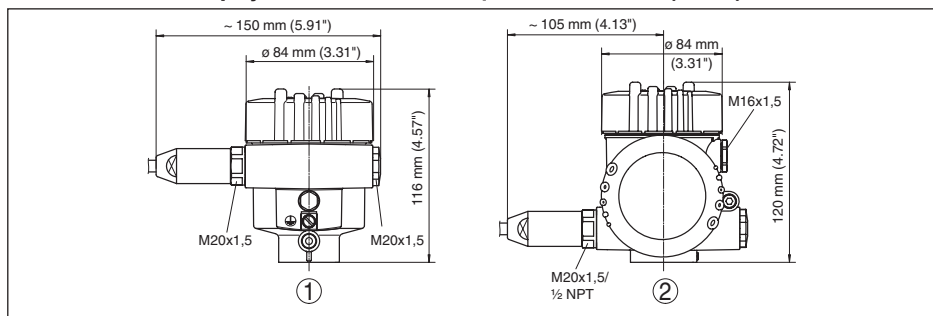
Рис. 64: Корпуса в исполнении IP 66/IP 68 (1 bar) - с установленным модулем индикации и настройки корпус выше на 9 mm/0.35 in
