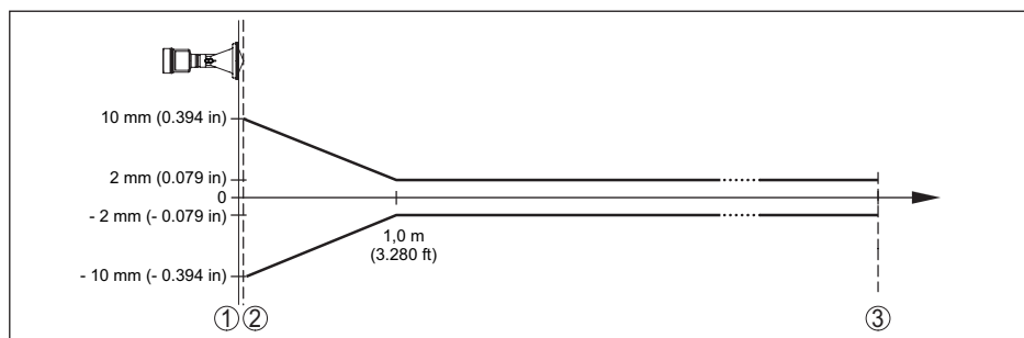
Рис. 52: Погрешность измерения при эталонных условиях
