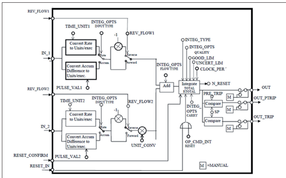
Рис. 59: Схема функционального блока Integrator
