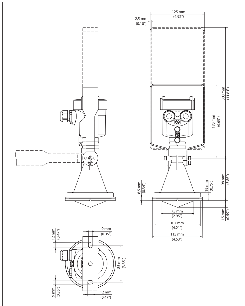
Рис. 67: VEGAPULS 67, монтажная скоба длиной 170 или 300 мм
