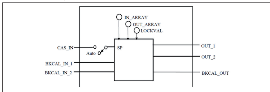
Рис. 57: Схема функционального блока Output Splitter
