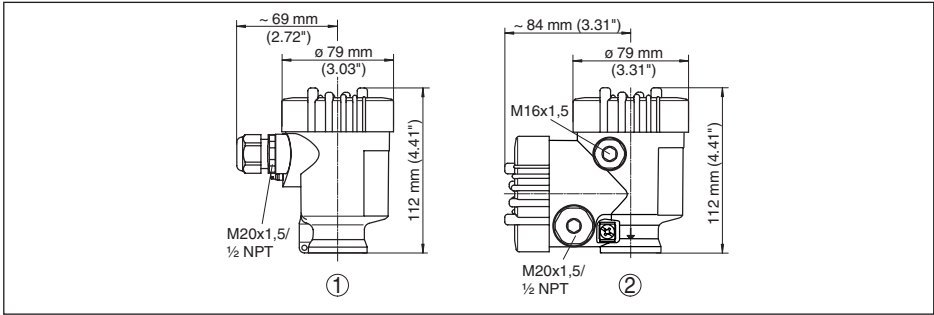
Рис. 62: Корпуса в исполнении IP 66/IP 68 (0,2 bar) - с установленным модулем индикации и настройки корпус выше на 9 mm/0.35 in
