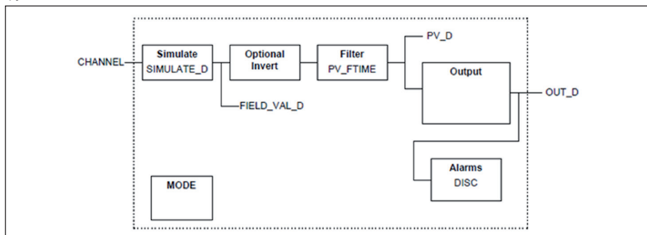
Рис. 55: Схема функционального блока Discret Input (DI)
