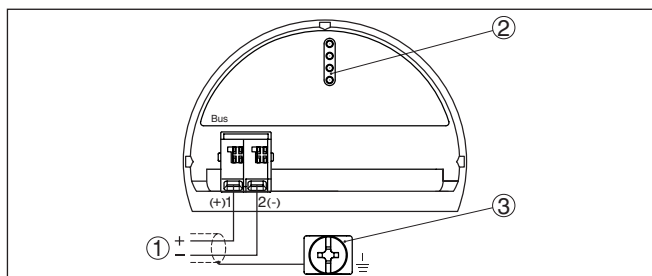
Рис. 29: Отсек подключения (двухкамерный корпус)
