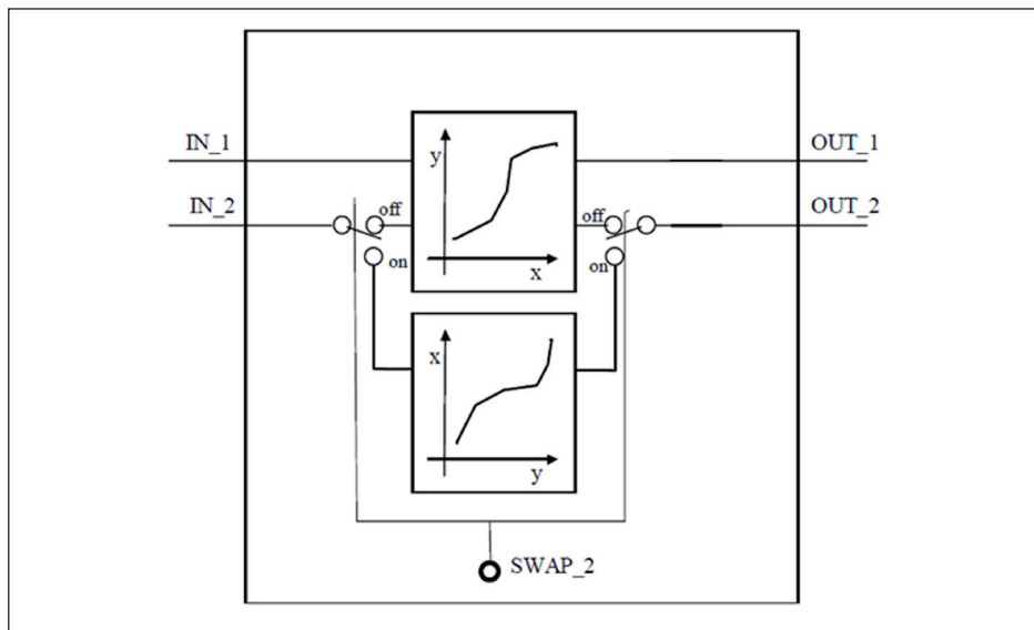
Рис. 58: Схема функционального блока Signal Characterizer
