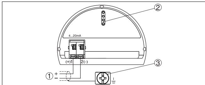
Рис. 30: Отсек подключения (двухкамерный корпус)
