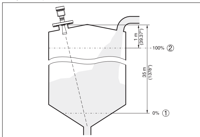
Рис. 39: Пример выполнения Установки Min./Max.
