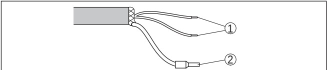
Рис. 35: Назначение проводов постоянно подключенного соединительного кабеля
