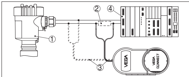
Рис. 41: Подключение ПК к сигнальному кабелю через HART
