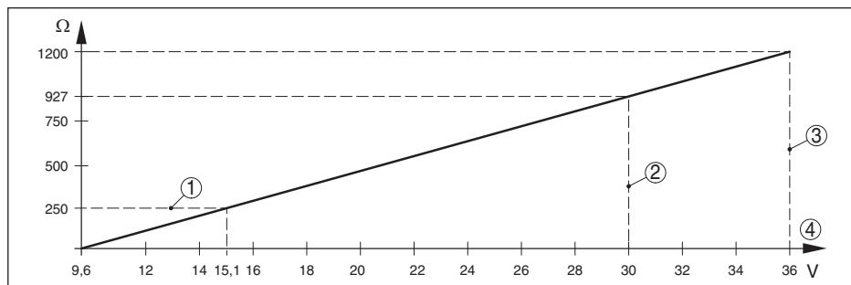
Рис. 55: Диаграмма напряжения
