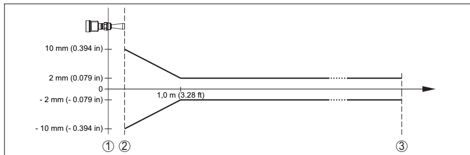
Рис. 54: Погрешность измерения при эталонных условиях
