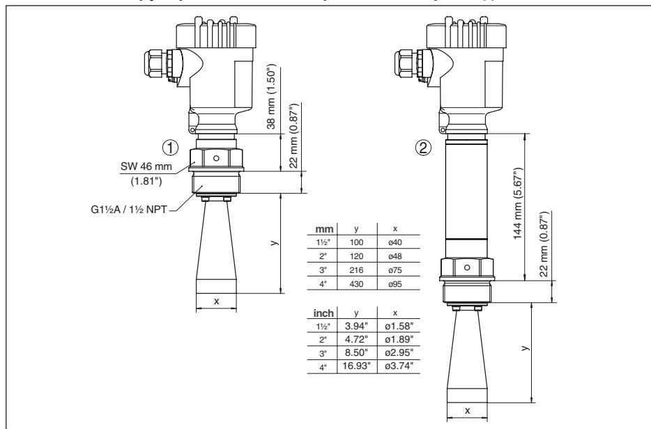
Рис. 61: VEGAPULS 68 с рупорной антенной и резьбовым присоединением
