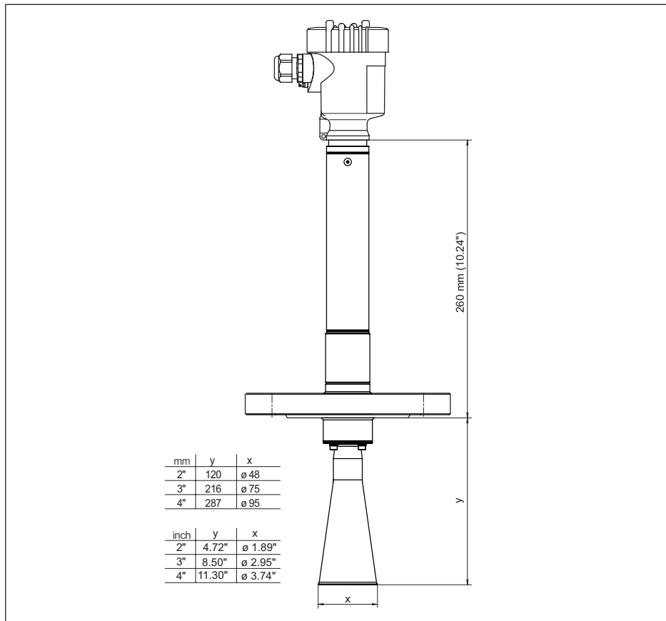
Рис. 63: VEGAPULS 68, с рупорной антенной и фланцевым присоединением, с температурной вставкой до 450 °C
