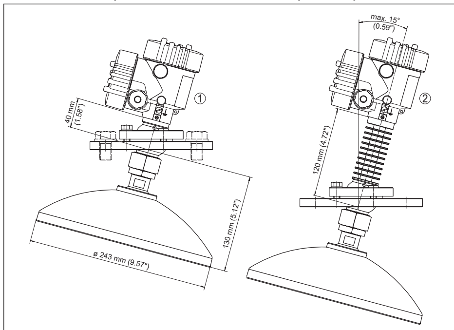
Рис. 55: VEGAPULS 68, с параболической антенной и поворотным креплением
