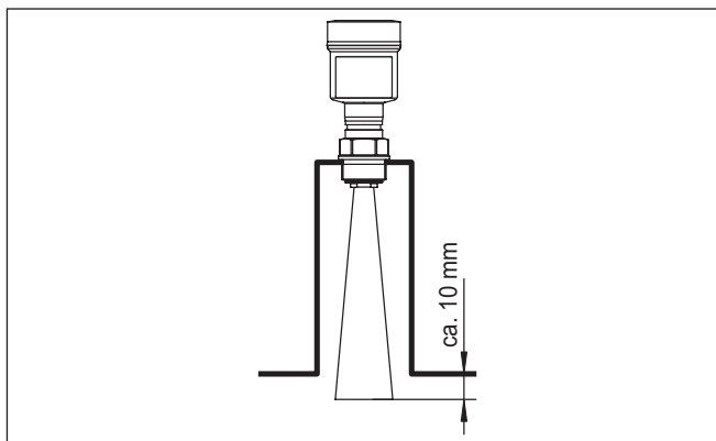
Рис. 11: Рекомендуемые размеры монтажного патрубка для прибора с рупорной антенной
