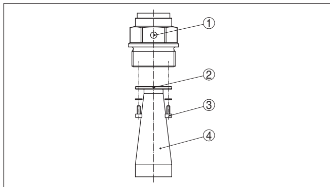
Рис. 5: Демонтаж рупорной антенны
