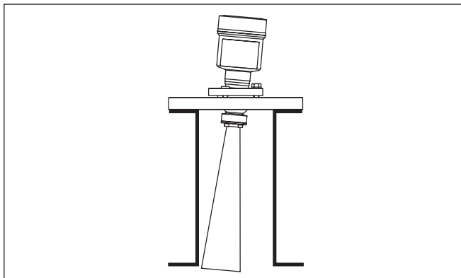
Рис. 13: Расстояние между антенной и патрубком для рупорной антенны
