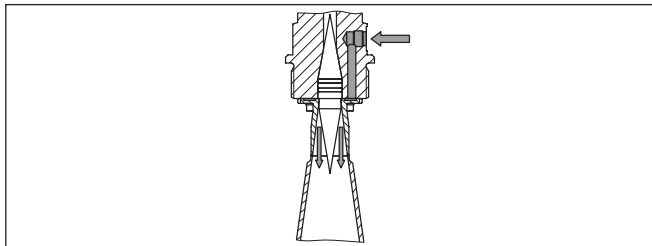
Рис. 25: Вход для подключения продувки рупорной антенны
