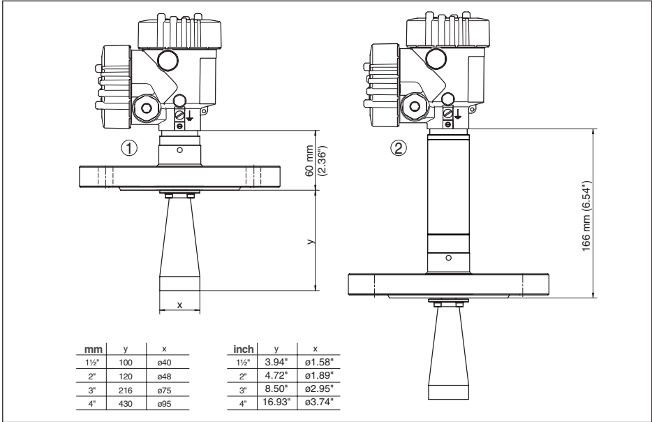
Рис. 52: VEGAPULS 68, с рупорной антенной и фланцевым присоединением
