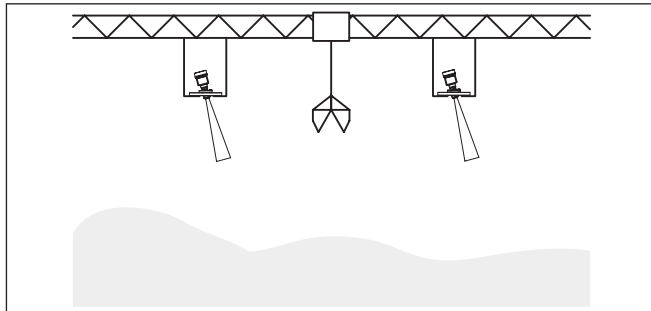
Рис. 20: Радарные датчики на кран-балке
