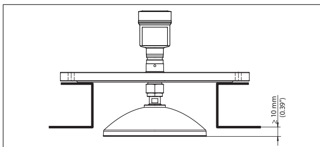
Рис. 12: Рекомендуемые размеры монтажного патрубка для прибора с параболической антенной
