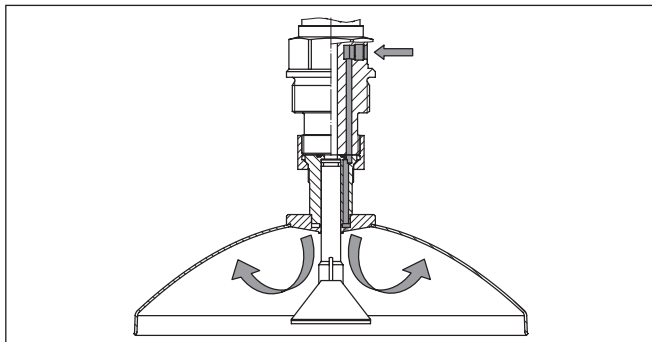
Рис. 26: Вход для подключения продувки параболической антенны
