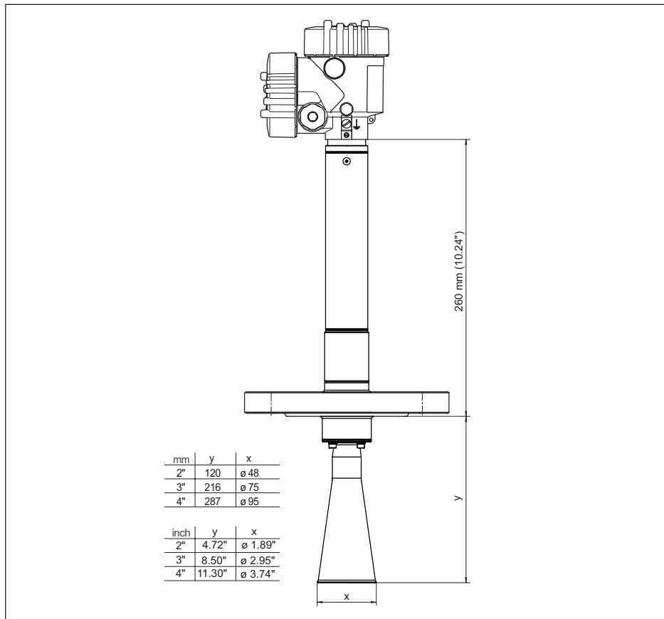
Рис. 53: VEGAPULS 68, с рупорной антенной и фланцевым присоединением, с температурной вставкой до 450 °C
