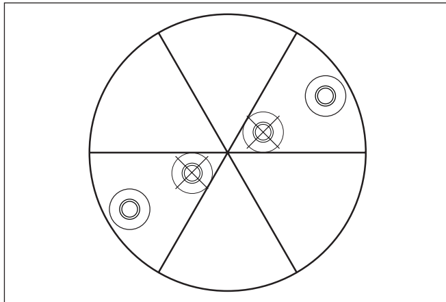
Рис. 23: Монтаж VEGAPULS 68 в многокамерном силосе
