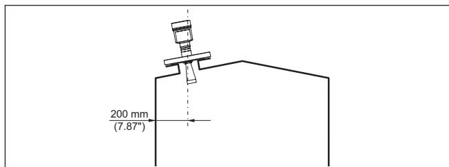
Рис. 8: Монтаж радарного датчика на крыше емкости
