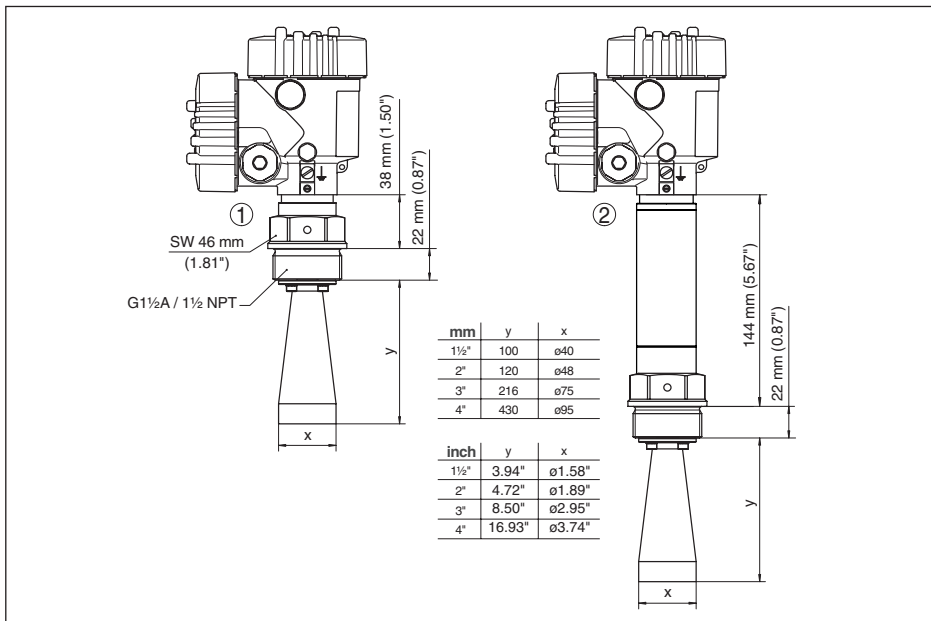
Рис. 51: VEGAPULS 68 с рупорной антенной и резьбовым присоединением
