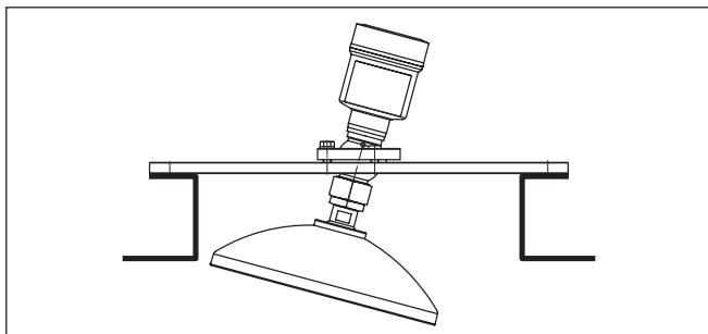
Рис. 14: Расстояние между антенной и патрубком для параболической антенны
