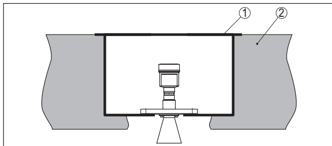
Рис. 22: Монтаж прибора в коробе под полом
