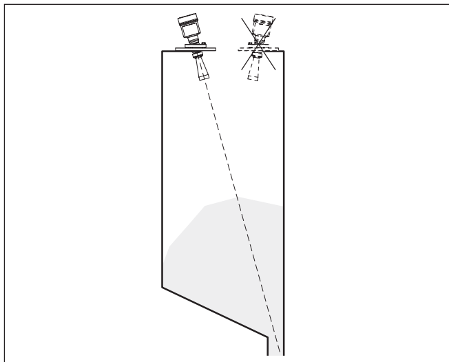
Рис. 24: Ориентация VEGAPULS 68 на выпускное отверстие в центре силоса
