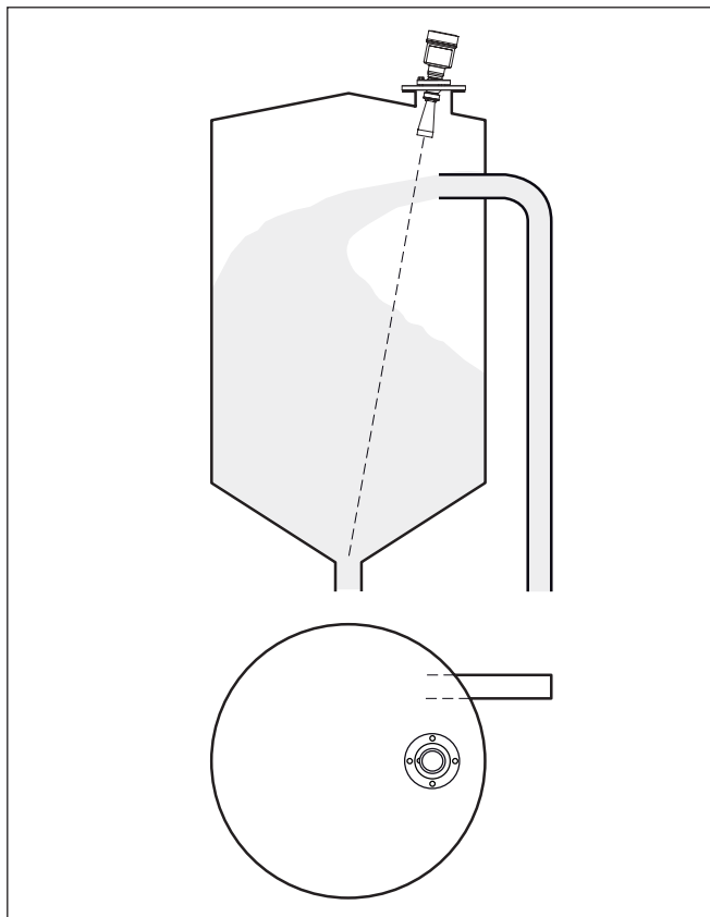
Рис. 10: Монтаж радарного датчика при втекающем продукте
