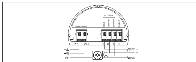
Рис. 2: Отсек подключения в двухкамерном корпусе в случае сетевого напряжения
