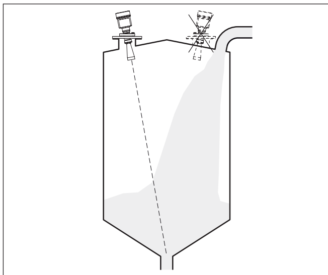
Рис. 9: Монтаж радарного датчика при втекающем продукте
