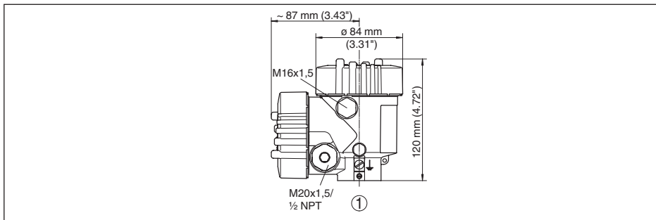
Рис. 50: Размеры корпуса - с установленным модулем индикации и настройки корпус выше на 9 мм (0.35 in)
