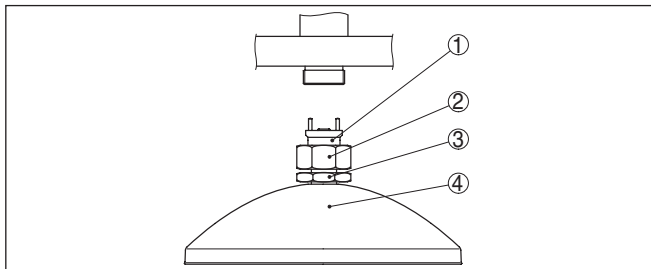
Рис. 6: Демонтаж параболической антенны
