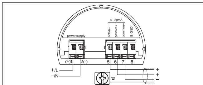
Рис. 30: Отсек подключения в двухкамерном корпусе в случае малого напряжения
