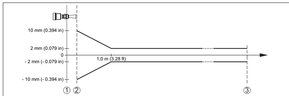
Рис. 49: Погрешность измерения при эталонных условиях
