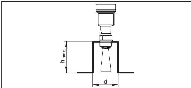
Рис. 15: Ориентировочные размеры патрубков
