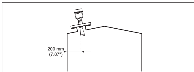
Рис. 7: Монтаж радарного датчика на крыше емкости
