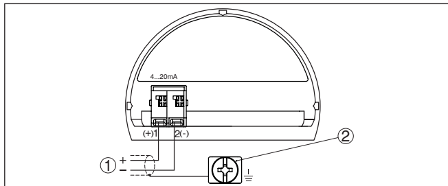
Рис. 29: Отсек подключения (двухкамерный корпус Ex d)
