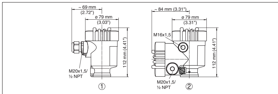
Рис. 52: Корпуса в исполнении IP 66/IP 68 (0,2 bar) - с установленным модулем индикации и настройки корпус выше на 9 мм/0.35 in
