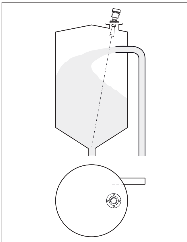
Рис. 9: Монтаж радарного датчика при втекающем продукте
