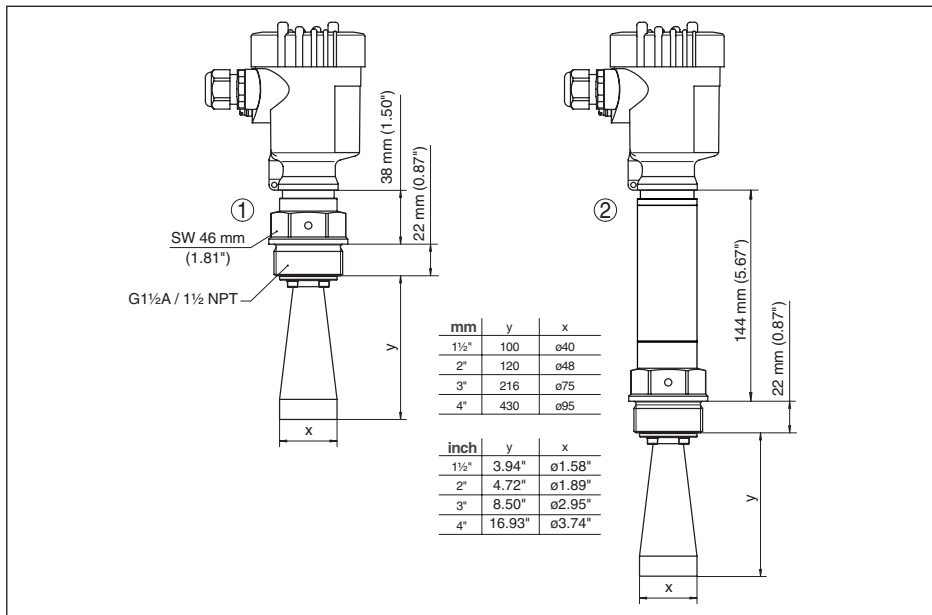
Рис. 57: VEGAPULS SR 68 с рупорной антенной и резьбовым присоединением
