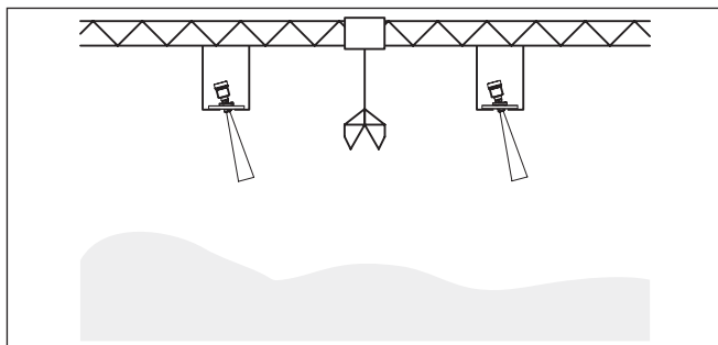
Рис. 17: Радарные датчики на кран-балке
