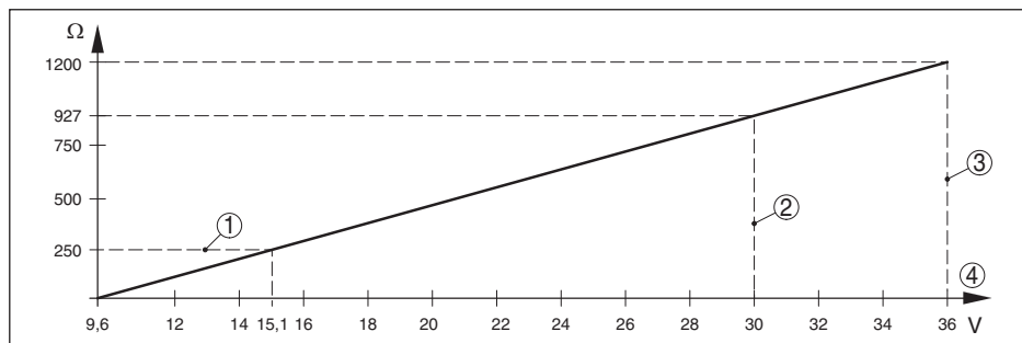
Рис. 51: Диаграмма напряжения
