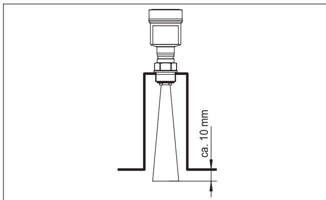
Рис. 10: Рекомендуемые размеры монтажного патрубка для прибора с рупорной антенной
