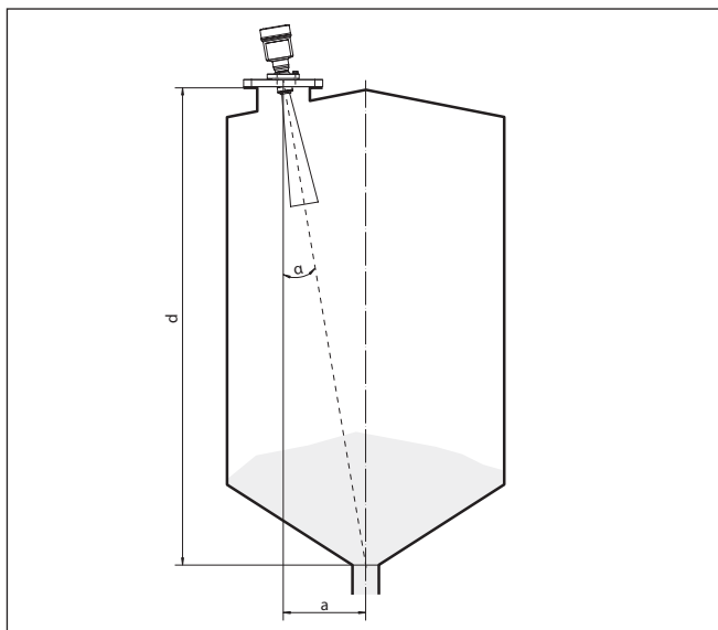
Рис. 14: Рекомендация по монтажу VEGAPULS SR 68 с наклоном
