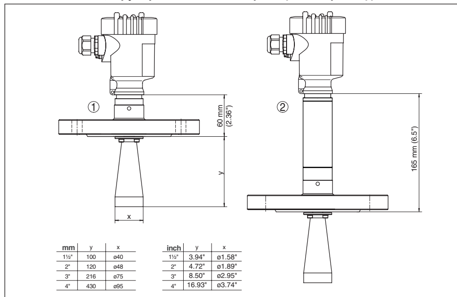
Рис. 58: VEGAPULS SR 68, с рупорной антенной и фланцевым присоединением
