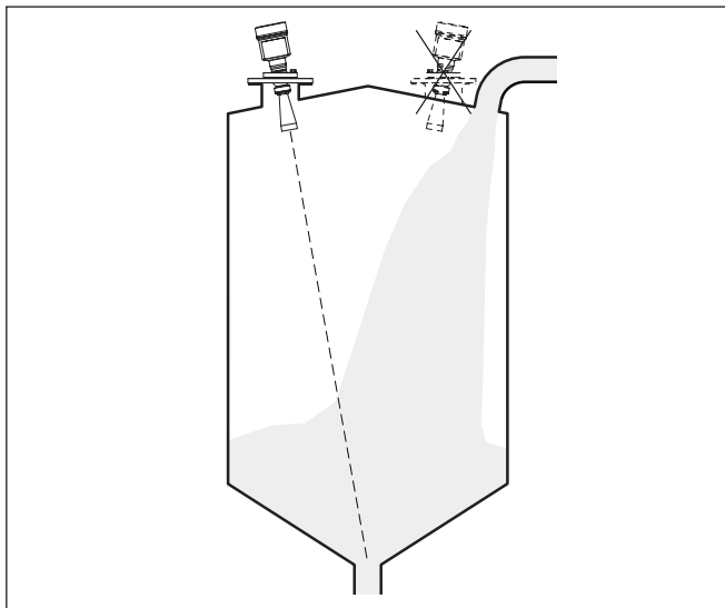
Рис. 8: Монтаж радарного датчика при втекающем продукте
