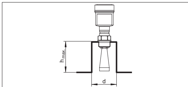
Рис. 12: Ориентировочные размеры патрубков
