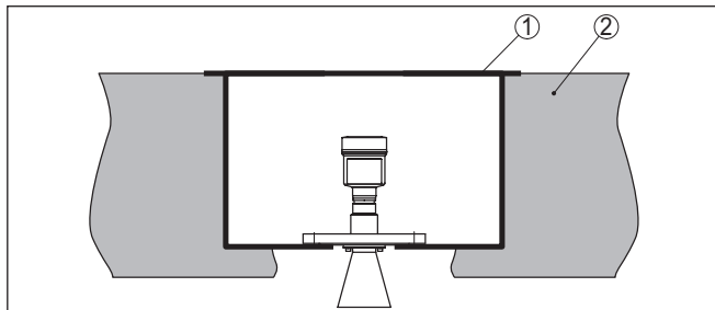
Рис. 19: Монтаж прибора в коробе под полом
