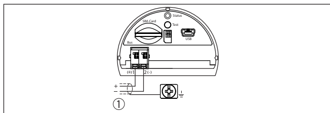
Рис. 27: Подключение модуля мобильной связи к питанию
