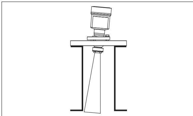
Рис. 11: Расстояние между антенной и патрубком для рупорной антенны
