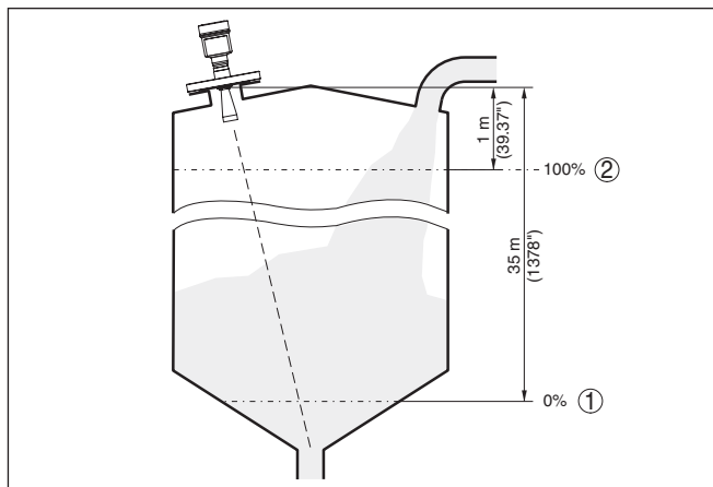
Рис. 35: Пример выполнения Установки Min./Max.
