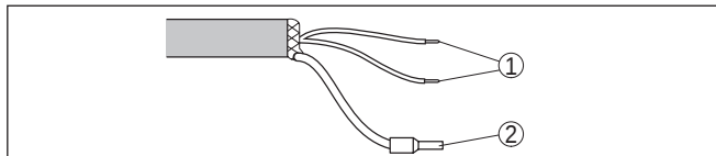
Рис. 31: Назначение проводов постоянно подключенного соединительного кабеля
