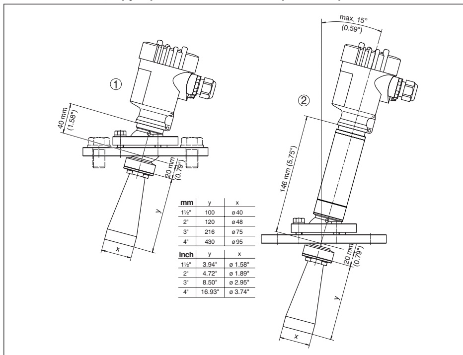
Рис. 59: VEGAPULS SR 68, с рупорной антенной и поворотным креплением
