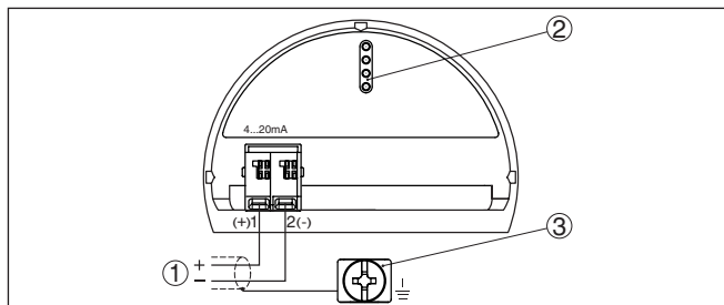
Рис. 26: Отсек подключения (двухкамерный корпус)
