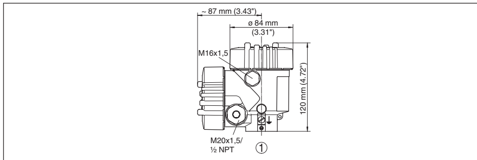
Рис. 46: Размеры корпуса - с установленным модулем индикации и настройки корпус выше на 9 мм (0.35 in)
