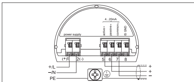
Рис. 25: Отсек подключения в двухкамерном корпусе в случае сетевого напряжения
