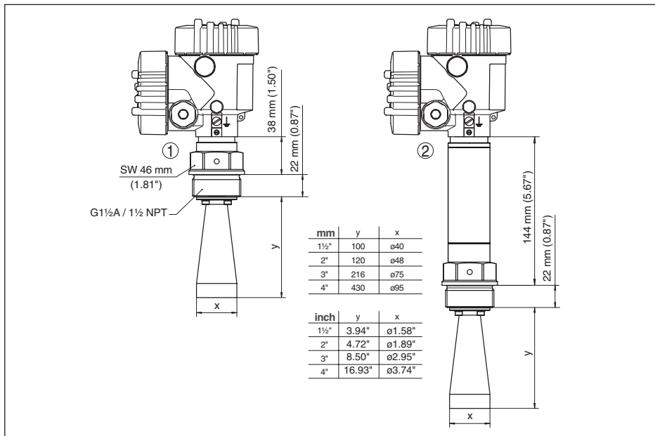
Рис. 47: VEGAPULS SR 68 с рупорной антенной и резьбовым присоединением
