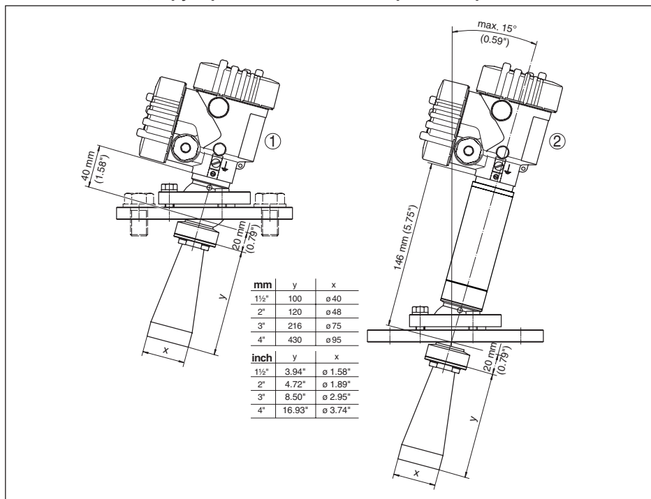
Рис. 49: VEGAPULS SR 68, с рупорной антенной и поворотным креплением
