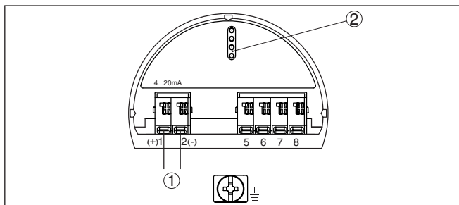
Рис. 24: Отсек электроники (двухкамерный корпус)
