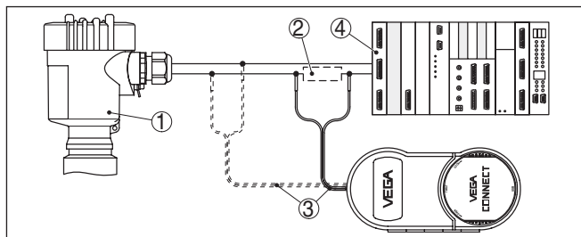
Рис. 32: Подключение ПК к сигнальному кабелю через HART
