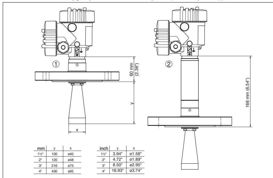
Рис. 48: VEGAPULS SR 68, с рупорной антенной и фланцевым присоединением
