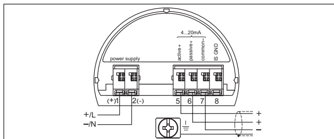
Рис. 26: Отсек подключения в двухкамерном корпусе в случае малого напряжения
