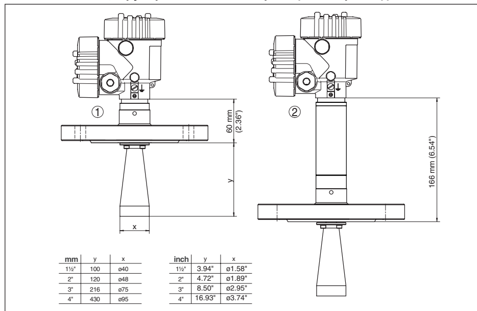
Рис. 55: VEGAPULS SR 68, с рупорной антенной и фланцевым присоединением
