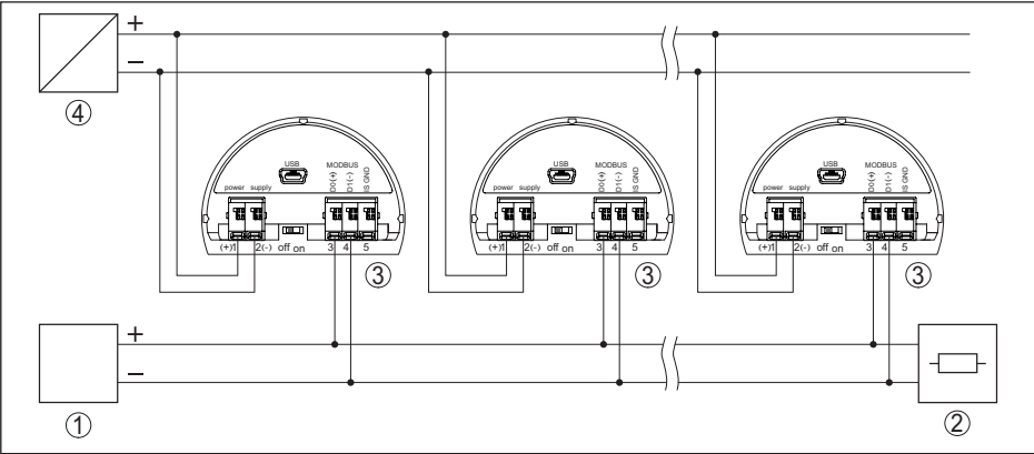
Рис. 47: Архитектура шины Modbus
