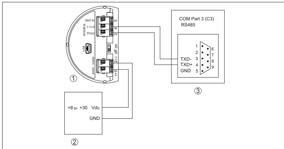
Рис. 52: Подключение VEGAPULS SR 68 к RTU ScadaPack
