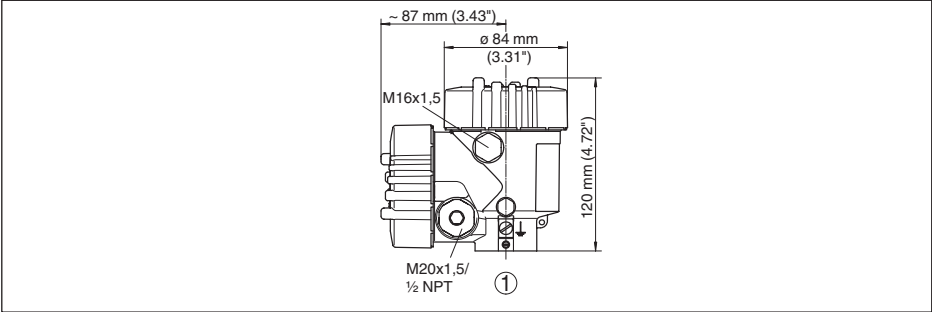
Рис. 53: Размеры корпуса - с установленным модулем индикации и настройки корпус выше на 9 мм (0.35 in)
