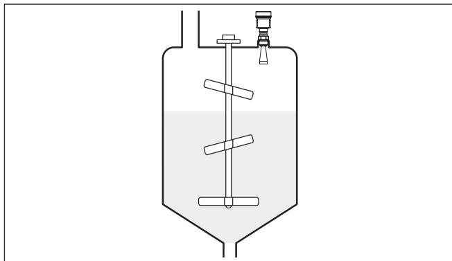
Рис. 17: Мешалки
