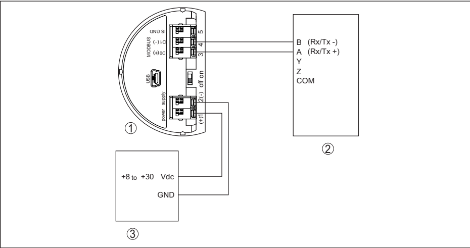
Рис. 48: Подключение VEGAPULS SR 68 к RTU Fisher ROC 809
