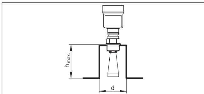
Рис. 13: Ориентировочные размеры патрубков
