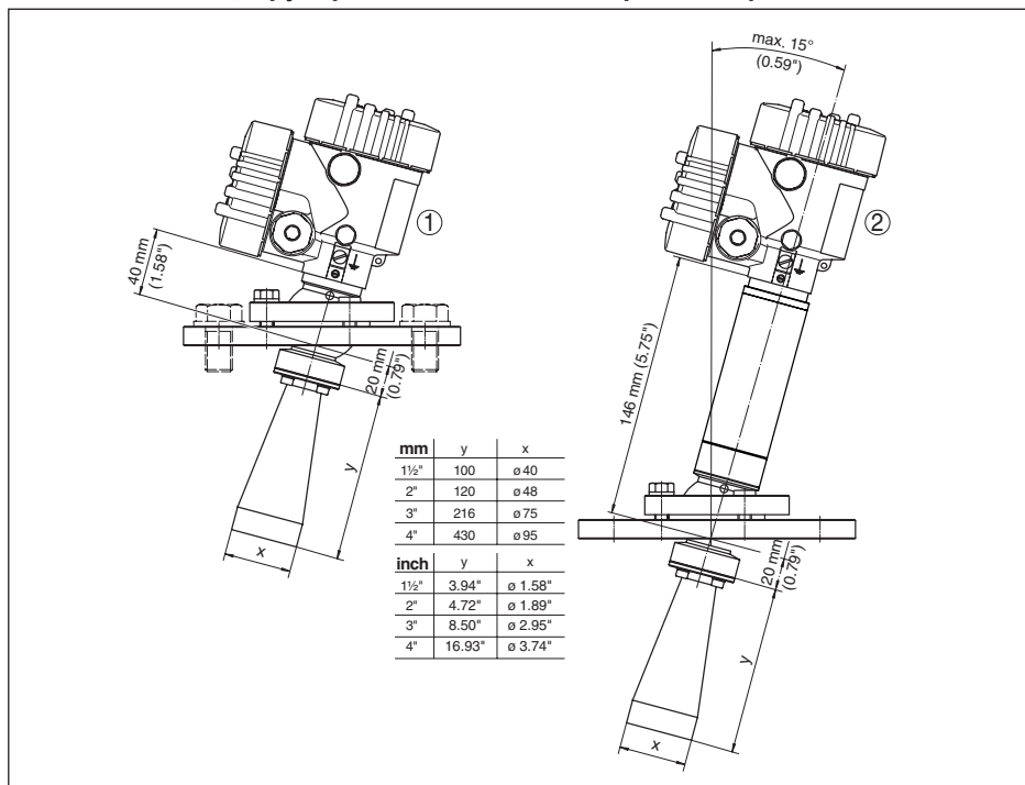
Рис. 56: VEGAPULS SR 68, с рупорной антенной и поворотным креплением
