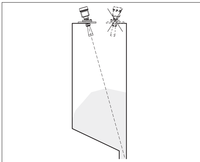
Рис. 22: Ориентация VEGAPULS SR 68 на выпускное отверстие в центре силоса
