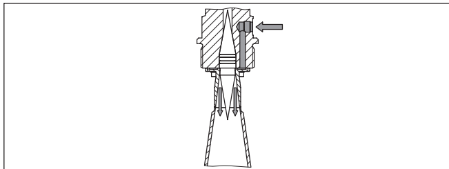
Рис. 23: Вход для подключения продувки рупорной антенны
