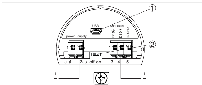
Рис. 27: Отсек подключения
