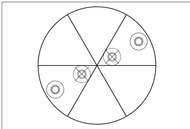
Рис. 21: Монтаж VEGAPULS SR 68 в многокамерном силосе
