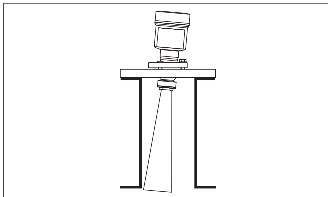
Рис. 12: Расстояние между антенной и патрубком для рупорной антенны
