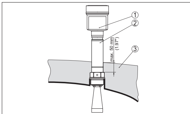
Рис. 19: Монтаж устройства на емкости с термоизоляцией
