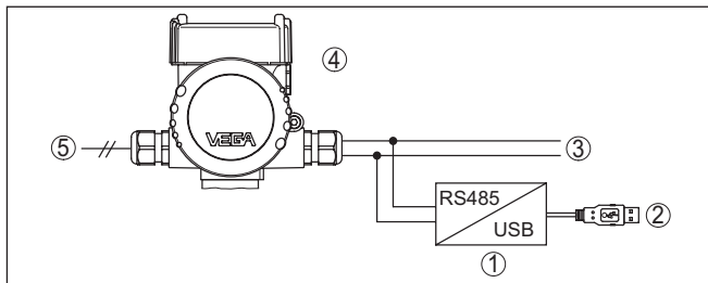
Рис. 33: Подключение ПК через интерфейсный адаптер к кабелю RS 485
