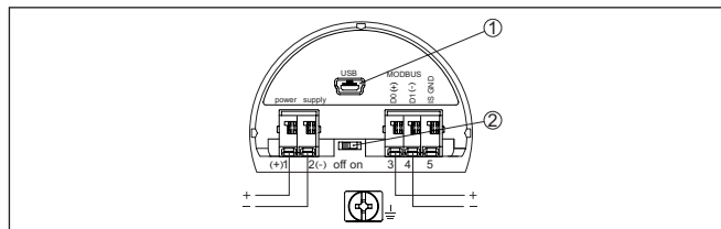
Рис. 2: Отсек подключения
