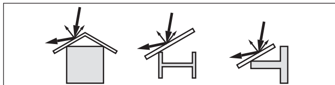
Рис. 16: Отражатели над конструкциями в емкости
