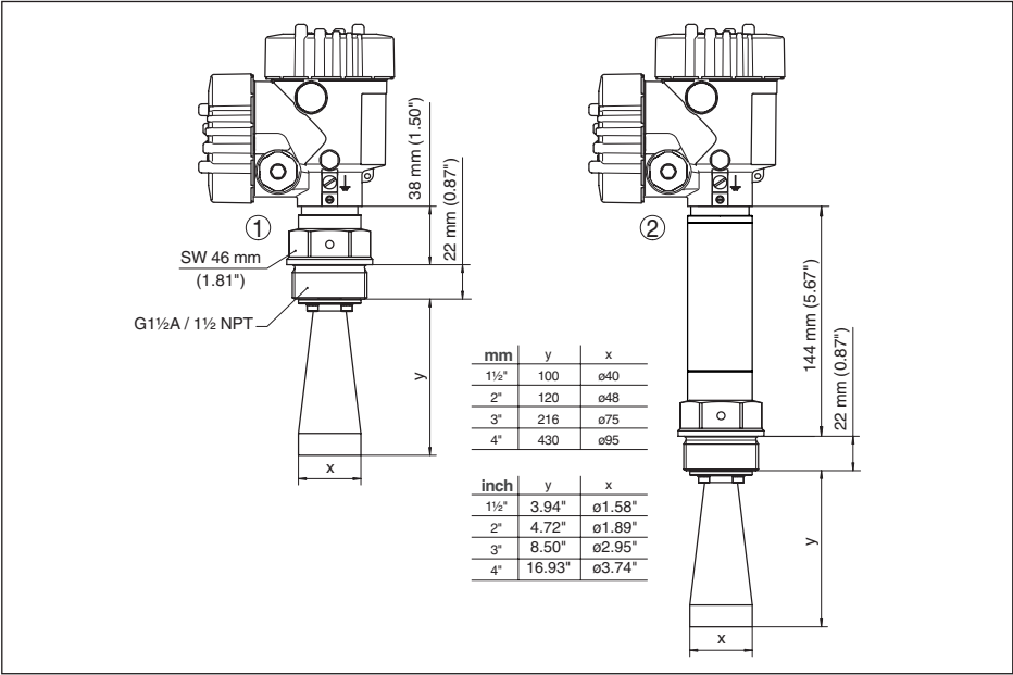
Рис. 54: VEGAPULS SR 68 с рупорной антенной и резьбовым присоединением
