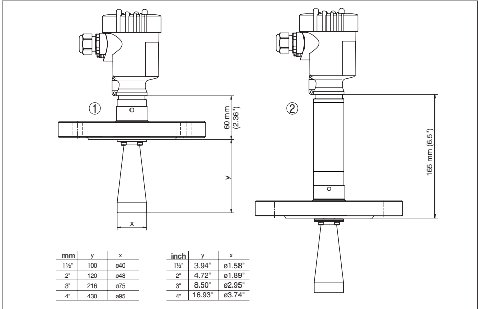
Рис. 59: VEGAPULS SR 68, с рупорной антенной и фланцевым присоединением
