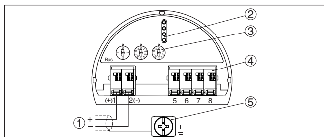
Рис. 24: Отсек электроники и подключения (однокамерный корпус)
