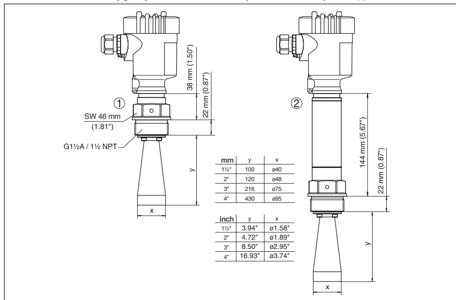
Рис. 58: VEGAPULS SR 68 с рупорной антенной и резьбовым присоединением
