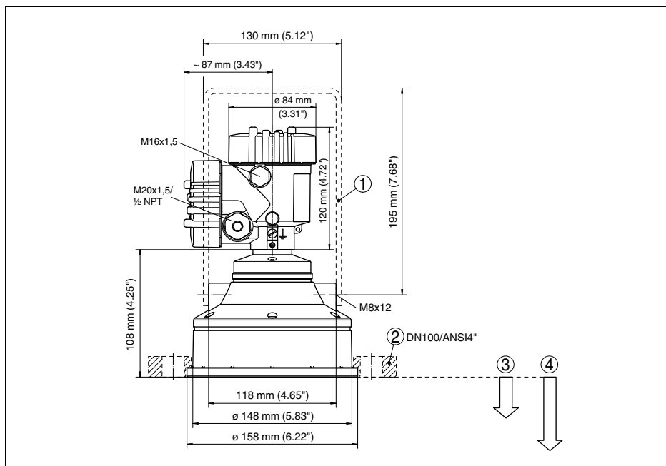
Рис. 26: VEGASON 63
