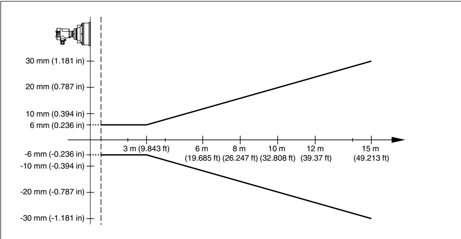
Рис. 25: Погрешность измерения VEGASON 63
