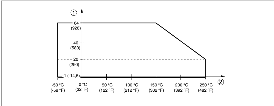
Рис. 33: Температура процесса - давление процесса при установке переключателя 0,5 г/см³ (переключатель чувствительности)
