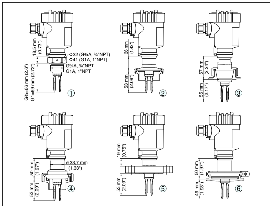
Рис. 35: VEGASWING 61
