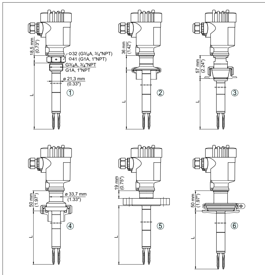
Рис. 48: VEGASWING 63
