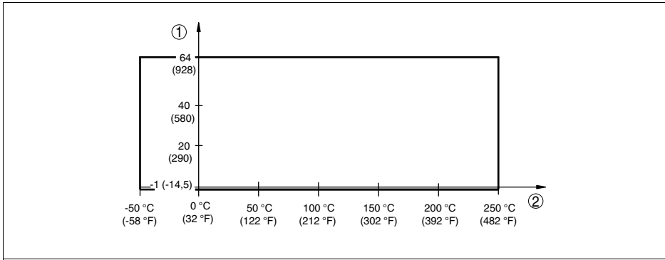
Рис. 44: Температура процесса - давление процесса при установке переключателя 0,7 г/см³ (переключатель чувствительности)
