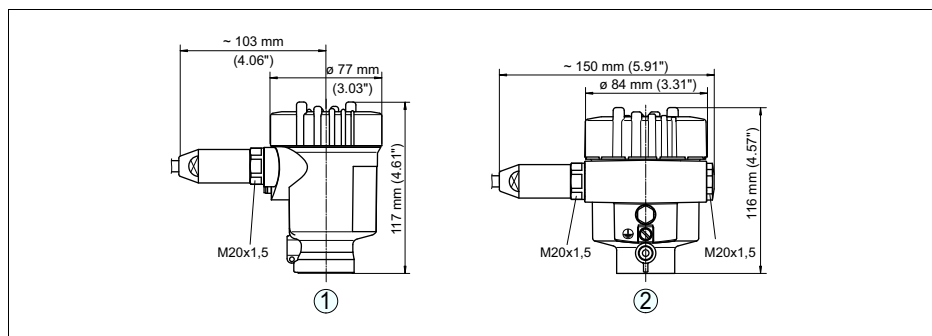
Рис. 47: Исполнения корпуса со степенью защиты IP 66/IP 68 (1 bar)
