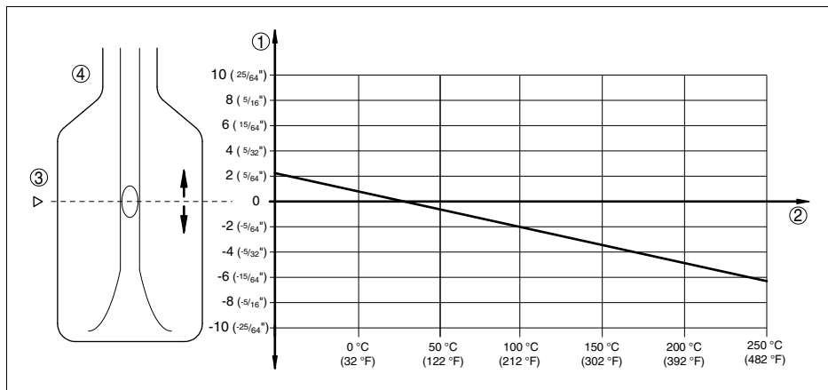
Рис. 40: Влияние температуры процесса на точку переключения
