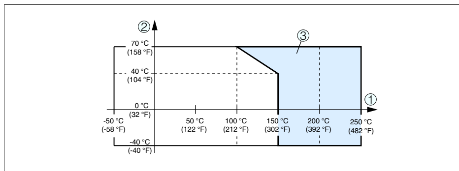
Рис. 43: Температура окружающей среды - Температура процесса
