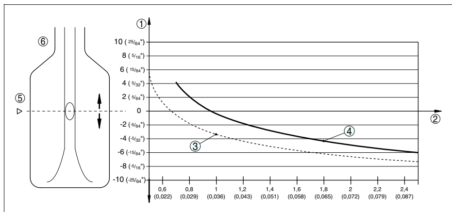
Рис. 41: Влияние плотности продукта на точку переключения
