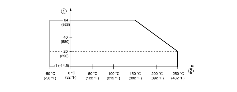
Рис. 45: Температура процесса - давление процесса при установке переключателя 0,5 г/см³ (переключатель чувствительности)
