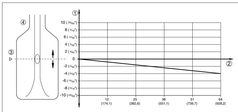
Рис. 42: Влияние давления процесса на точку переключения
