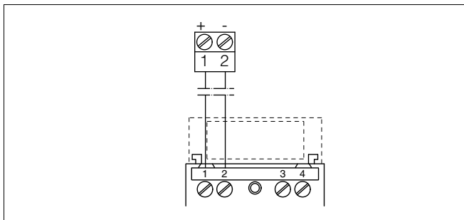
Рис. 12: Схема подключения (однокамерный корпус)
