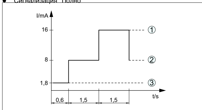
Рис. 29: Схема функциональной проверки
