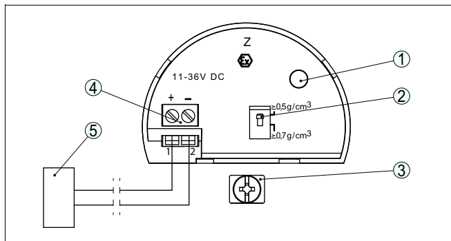
Рис. 11: Отсек электроники и подключения
