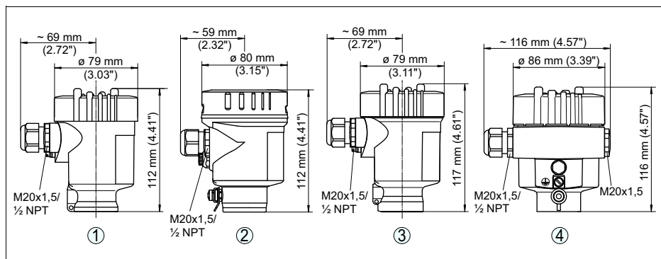
Рис. 46: Исполнения корпуса со степенью защиты IP 66/IP 67 и IP 66/IP 68; 0,2 bar
