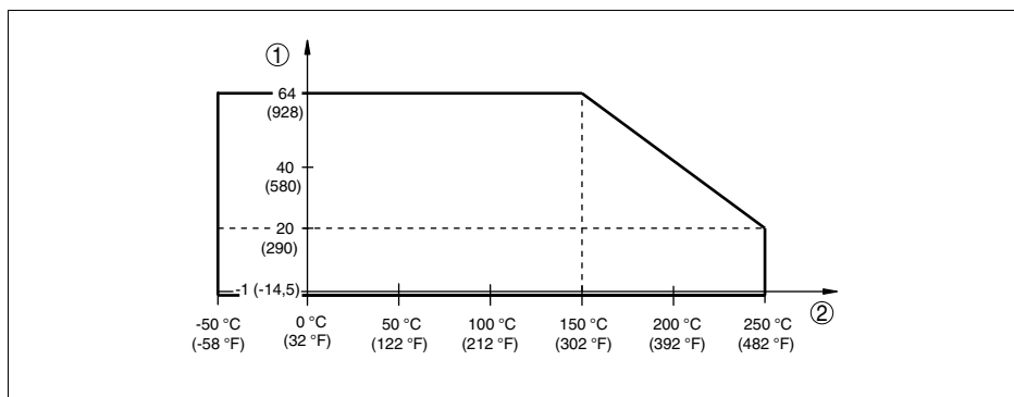
Рис. 29: Температура процесса - давление процесса при установке переключателя 0,5 г/см³ (переключатель чувствительности)
