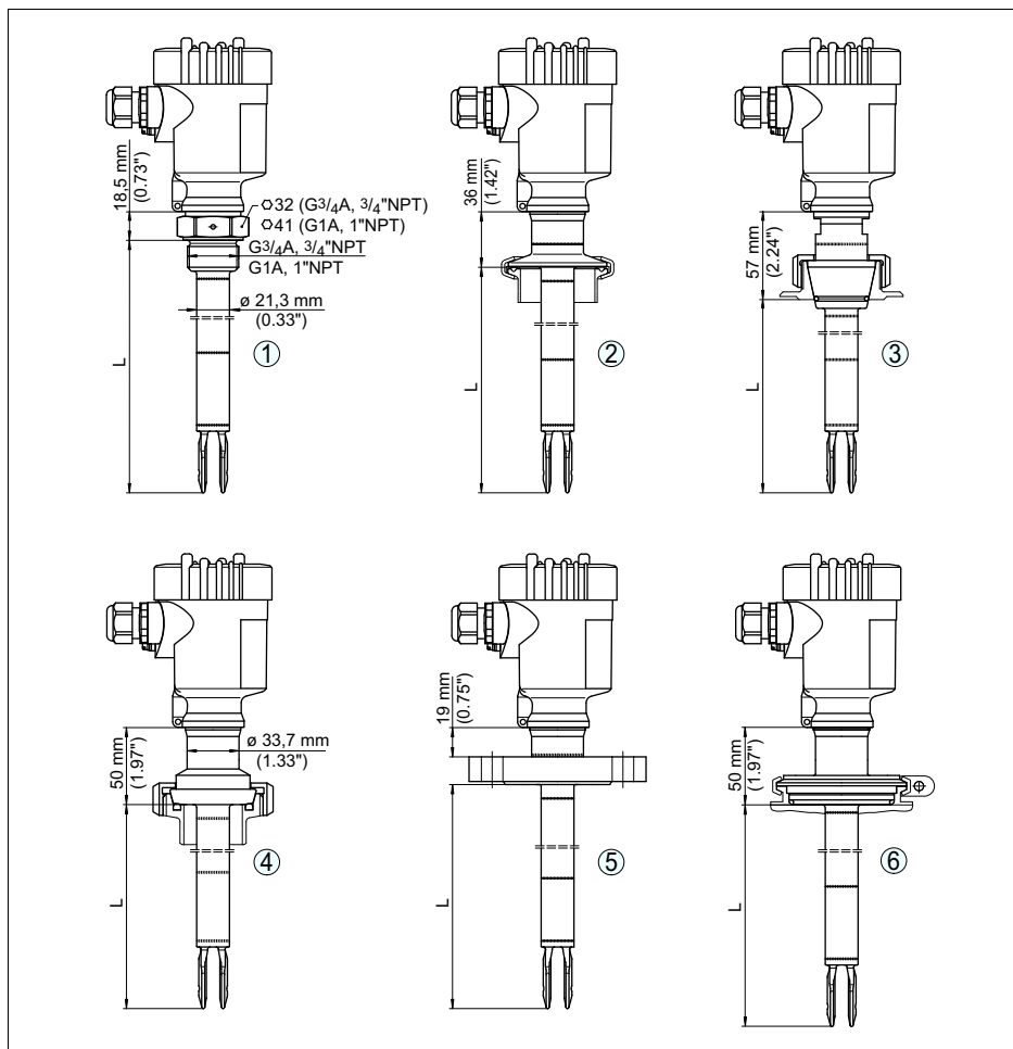
Рис. 34: VEGASWING 63
