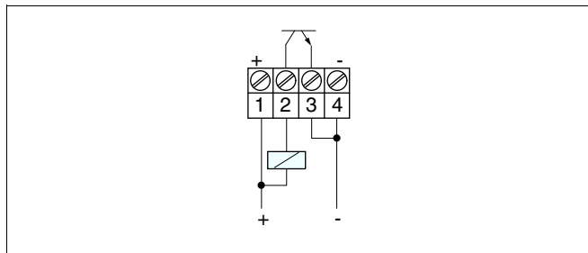
Рис. 12: Состояние NPN
