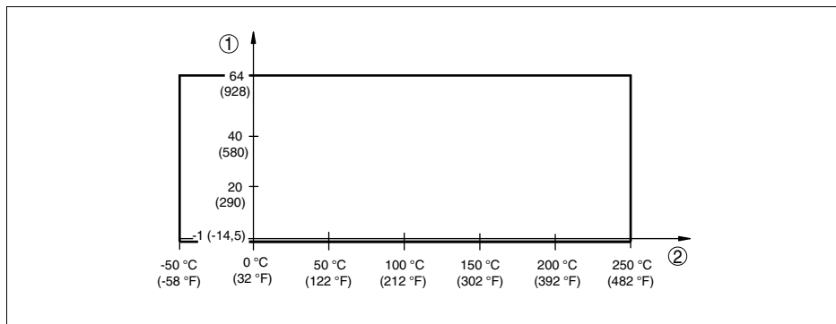
Рис. 30: Температура процесса - давление процесса при установке переключателя 0,7 г/см³ (переключатель чувствительности)
