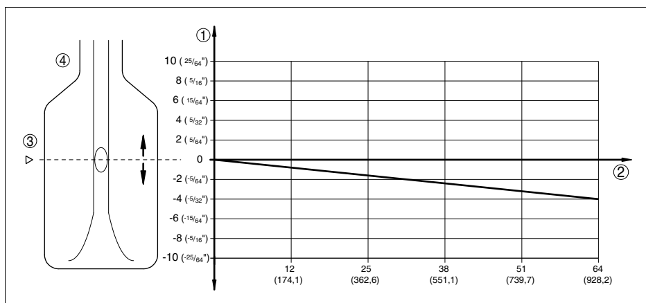
Рис. 28: Влияние давления процесса на точку переключения
