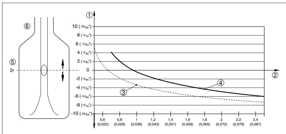
Рис. 27: Влияние плотности продукта на точку переключения
