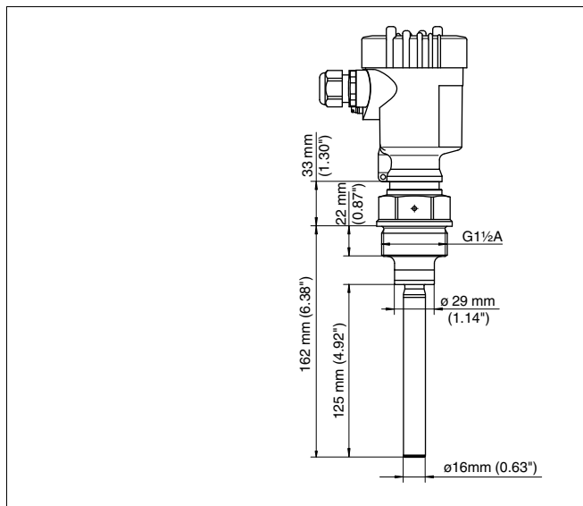
Рис. 33: VEGAVIB 61, резьбовое исполнение G1½ A (DIN ISO 228/1)
