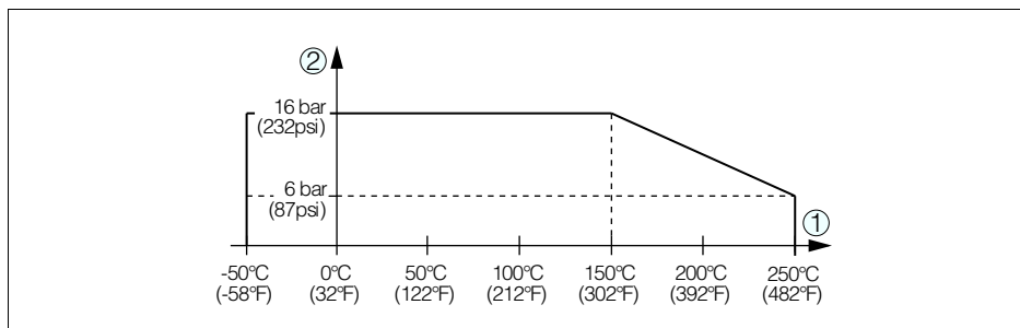
Рис. 29: Давление процесса - температура процесса
