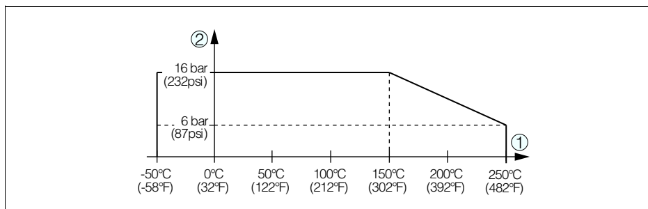
Рис. 31: Давление процесса - температура процесса
