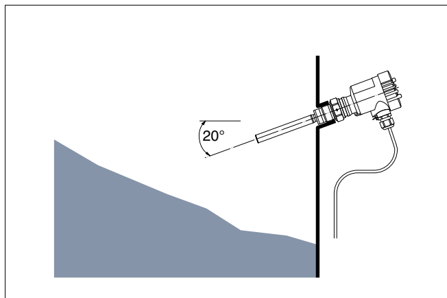
Рис. 6: Горизонтальный монтаж
