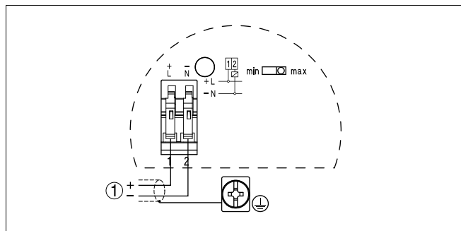
Рис. 9: Схема подключения
