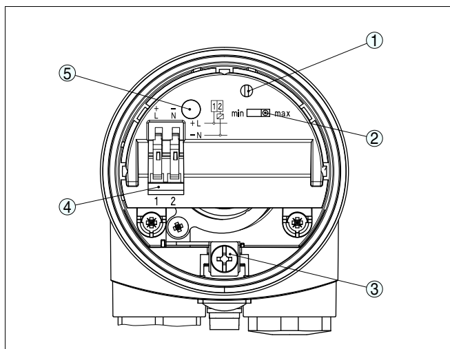
Рис. 10: Отсек электроники и подключения - бесконтактный переключатель
