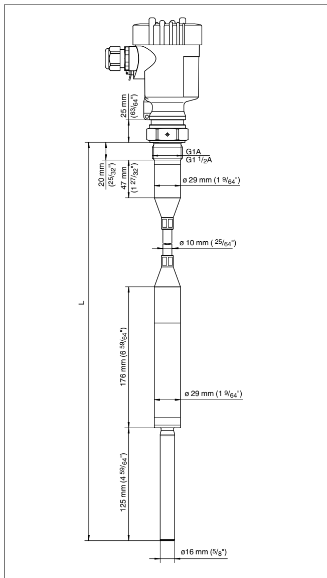
Рис. 30: VEGAVIB 62 с несущим тросом FEP
