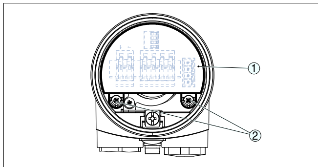
Рис. 27: Крепежные винты
