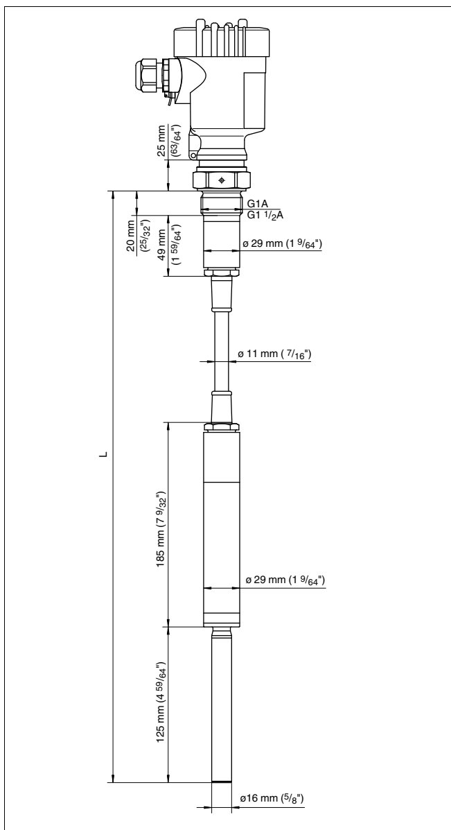
Рис. 29: VEGAVIB 62 с несущим тросом PUR
