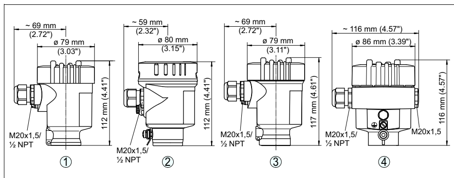
Рис. 25: Исполнения корпуса со степенью защиты IP 66/IP 67 и IP 66/IP 68; 0,2 bar
