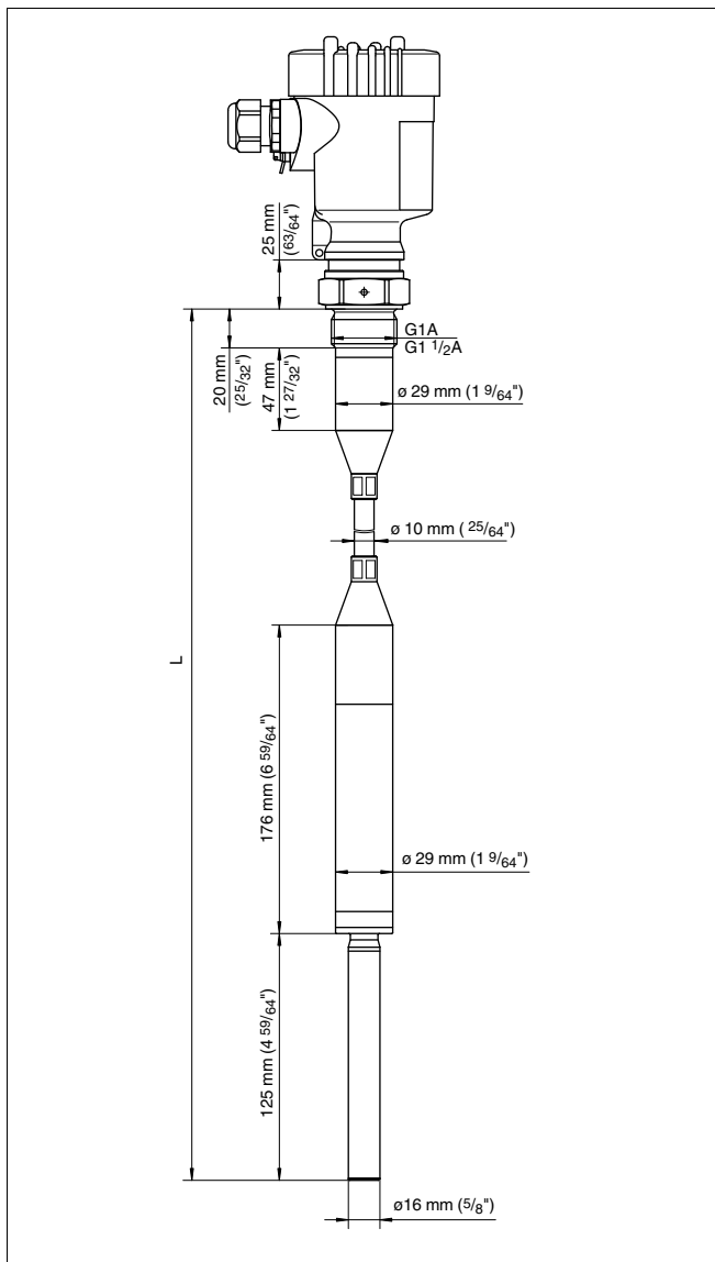
Рис. 28: VEGAVIB 62 с несущим тросом FEP
