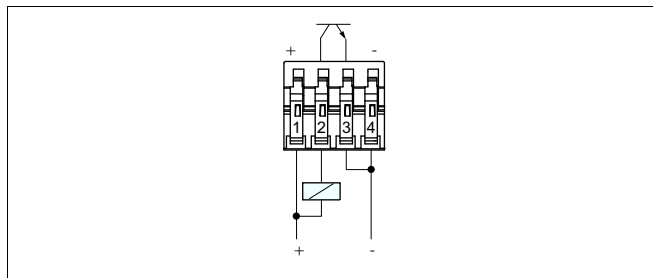
Рис. 10: Состояние NPN
