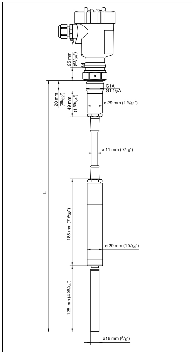
Рис. 27: VEGAVIB 62 с несущим тросом PUR
