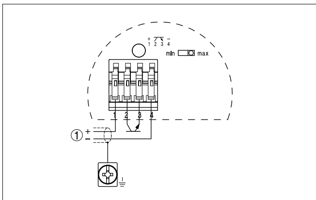
Рис. 9: Схема подключения
