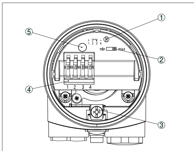
Рис. 13: Отсек электроники и подключения - транзисторный выход
