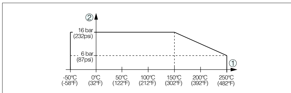
Рис. 28: Давление процесса - температура процесса
