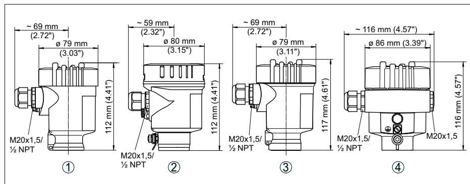
Рис. 30: Исполнения корпуса
