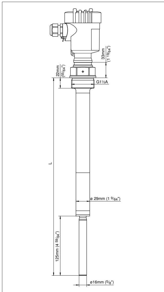
Рис. 32: VEGAVIB 63, резьбовое исполнение G1 1/2 A (DIN ISO 228/1)
