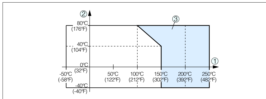
Рис. 31: Температура окружающей среды - Температура процесса
