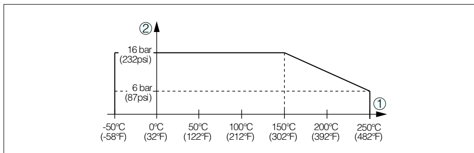
Рис. 30: Давление процесса - температура процесса
