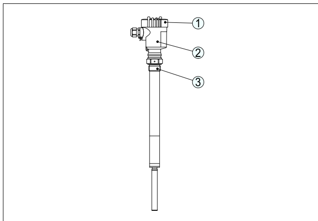
Рис. 1: VEGAVIB 63 - с пластиковым корпусом
