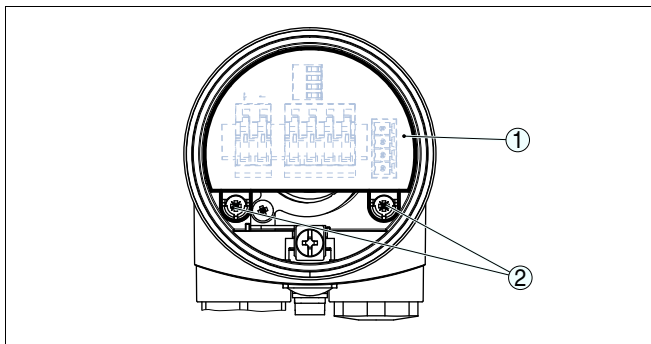
Рис. 29: Крепежные винты
