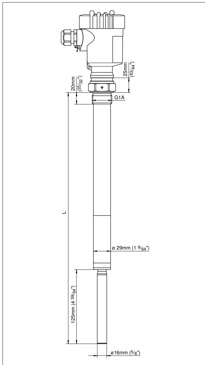
Рис. 34: VEGAVIB 63, резьбовое исполнение G1 A (DIN ISO 228/1)
