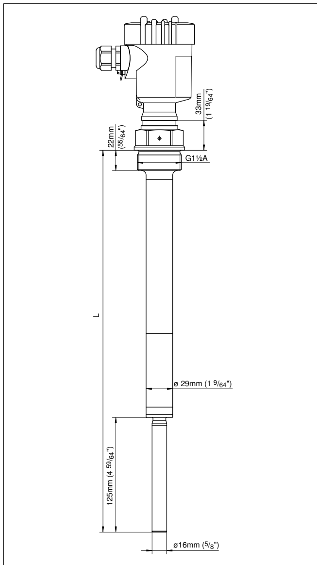
Рис. 30: VEGAVIB 63, резьбовое исполнение G1 1/2 A (DIN ISO 228/1)
