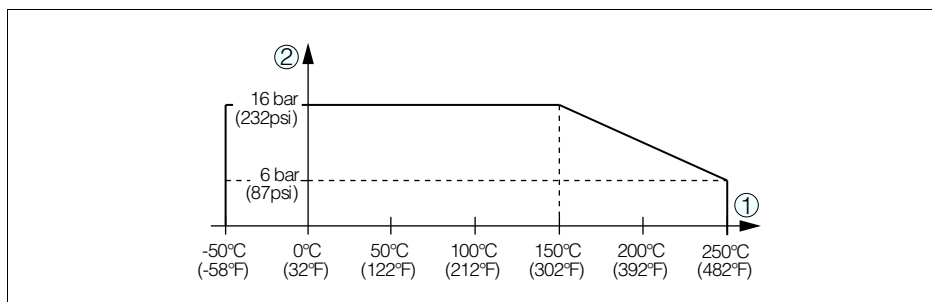
Рис. 25: Давление процесса - температура процесса
