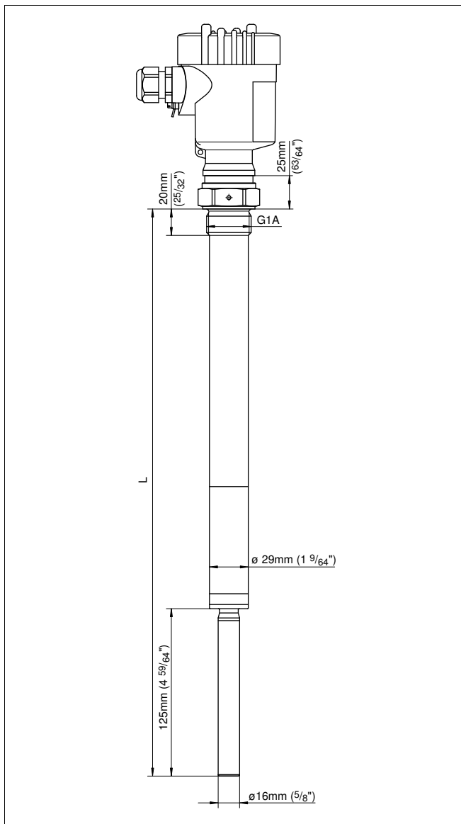
Рис. 29: VEGAVIB 63, резьбовое исполнение G1 A (DIN ISO 228/1)
