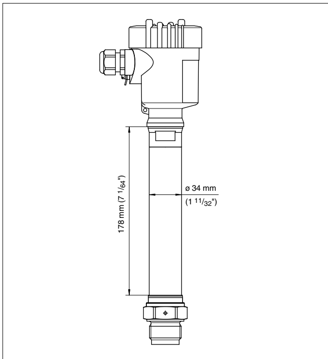
Рис. 31: Температурная вставка
