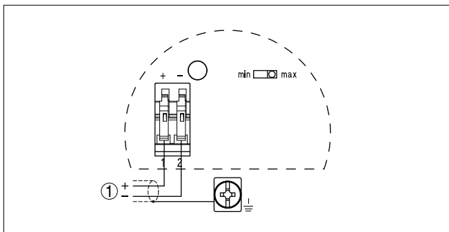
Рис. 10: Схема подключения
