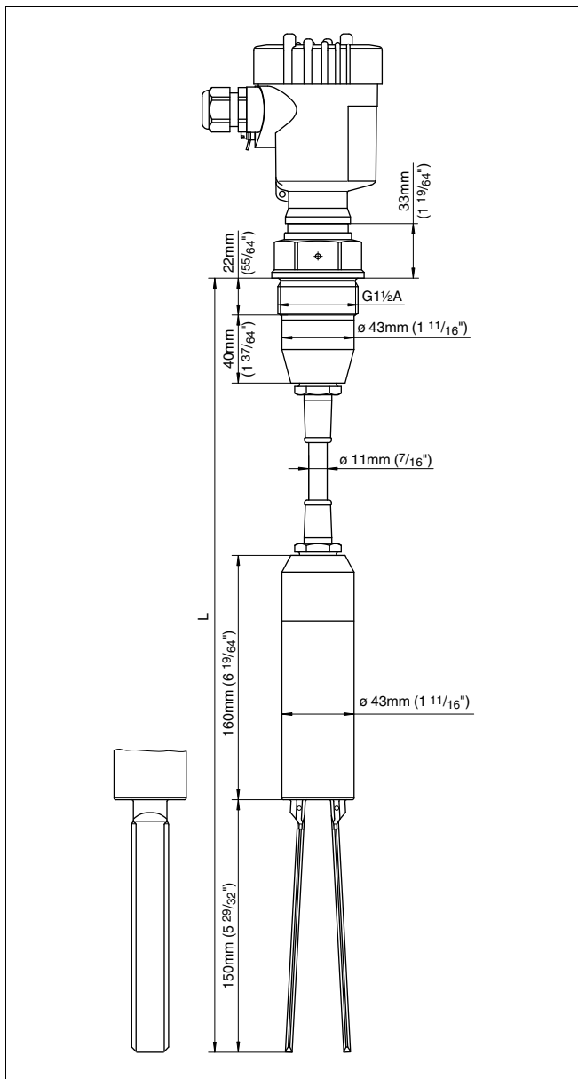
Рис. 50: VEGAWAVE 62 с несущим кабелем PUR, резьбовое исполнение G1½ A (DIN ISO 228/1)
