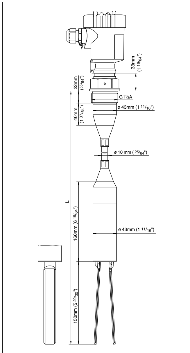
Рис. 51: VEGAWAVE 62 с несущим кабелем FEP, резьбовое исполнение G1\frac{1}{2}A (DIN ISO 228/1)
