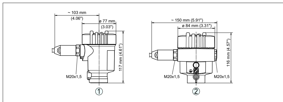
Рис. 49: Исполнения корпуса со степенью защиты IP 66/IP 68 (1 bar)
