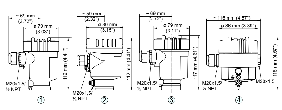
Рис. 48: Исполнения корпуса со степенью защиты IP 66/IP 67 и IP 66/IP 68; 0,2 bar
