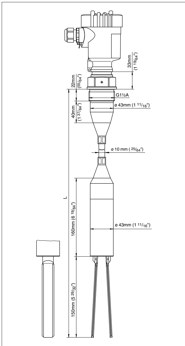
Рис. 34: VEGAWAVE 62 с несущим кабелем FEP, резьбовое исполнение G1 1/2 A (DIN ISO 228/1)
