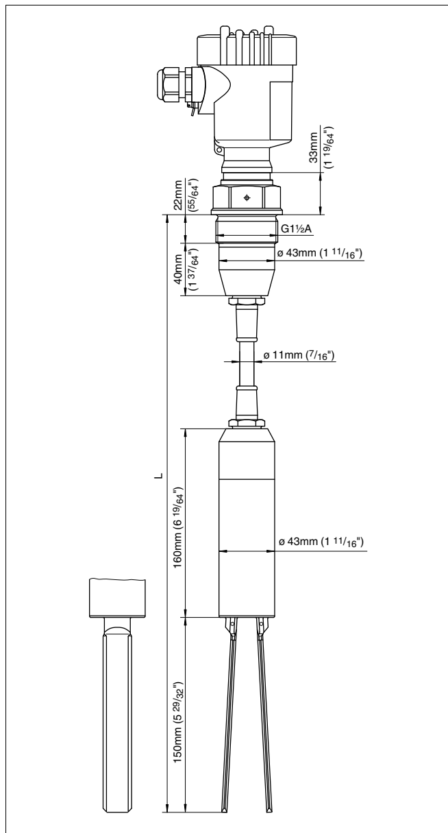
Рис. 33: VEGAWAVE 62 с несущим кабелем PUR, резьбовое исполнение G1½ A (DIN ISO 228/1)
