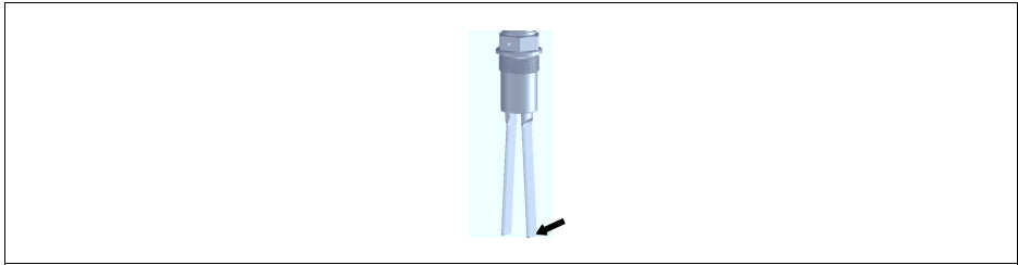
Рис. 31: Максимальная боковая нагрузка вдоль стороны вилки (к узкой стороне вилки)
