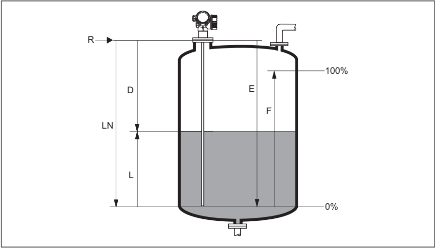
8 Параметры конфигурации для измерения уровня жидкостей
