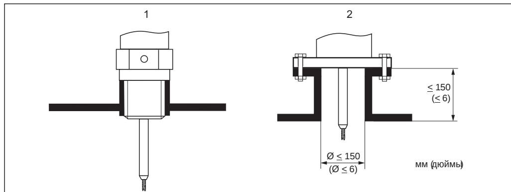
1 Монтаж в резьбовом соединении заподлицо к внутренней поверхности крыши силоса 2 Установка в патрубке
