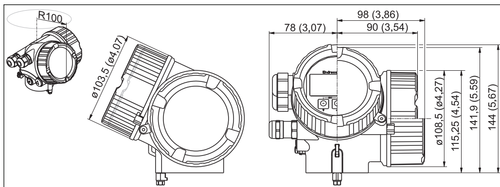
2 Корпус GT18 (316L); размеры в мм (дюймах)
