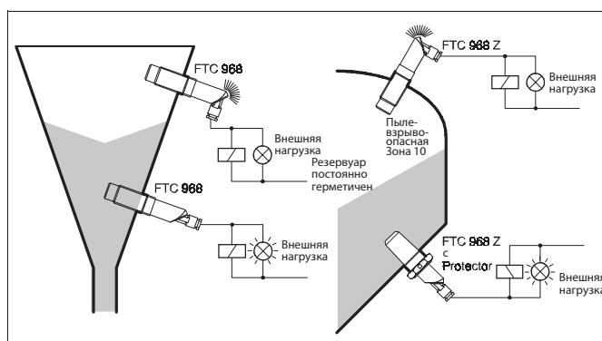
Рис. 1 Измерительная система
