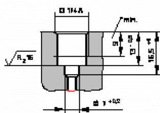
Уплотнение по DIN 16288
