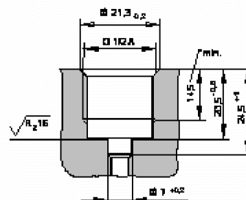
Уплотнение при помощи плоских уплотняющих элементов
